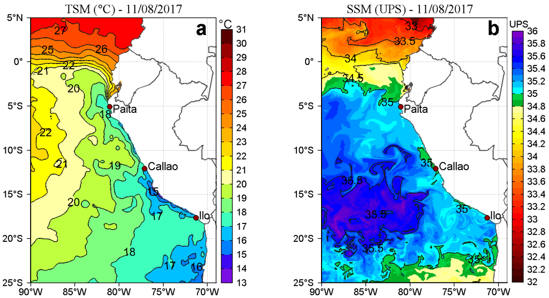
Figura 2. a) Temperatura superficial del mar ( ^{\circ}\text{C} ) y b) Salinidad superficial del mar (UPS) para el 11 de agosto respectivamente. Datos: OSTIA-UKMO-L4-GLOB-v2.0 (UK Met Office, 2012; Donlon et al, 2012) disponible en https://podaac.jpl.nasa.gov/dataset/OSTIA-UKMO-L4-GLOB-v2.0 para (a) y Hybrid Coordinate Ocean Model (HYCOM; Halliwell et al., 1998; 2000; Bleck, 2001) para (b). Procesamiento: LHF/AFIOF/DGIOCC/IMARPE.
