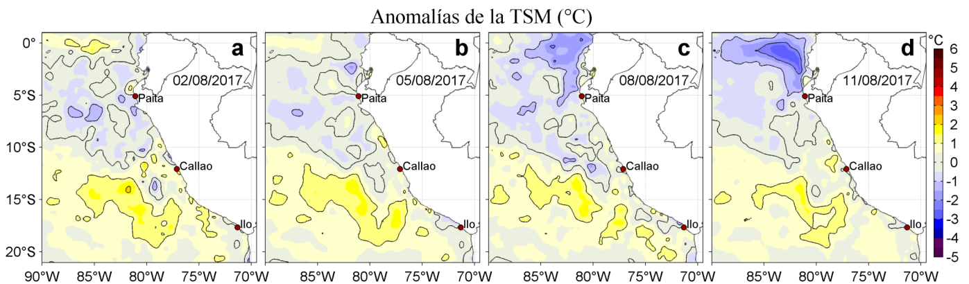
Figura 3. Anomalías de la Temperatura Superficial del Mar ( ^{\circ}\text{C} ) para los días: a) 02, b) 05, c) 08, y d) 11 de agosto de 2017. Las anomalías se calcularon respecto de la climatología para el periodo 2007-2016. Datos: OSTIA-UKMO-L4-GLOB-v2.0 (UK Met Office, 2012; Donlon et al, 2012). Procesamiento: LHF/AFIOF/DGIOCC/IMARPE.
