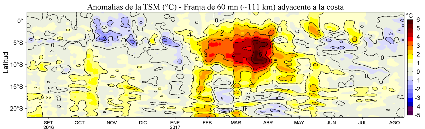
Figura 4. Variación promedio de las anomalías de la temperatura superficial del mar (°C) para una franja de 60 mn (~111 km) adyacente al litoral peruano para los últimos doce meses al 10 de agosto de 2017. Se distingue el calentamiento ocurrido de mediados de enero a fines de mayo de 2017 asociado con la presencia de El Niño Costero, evento que tuvo mayor impacto en la TSM (+5°C) en la segunda quincena de marzo. Datos: OSTIA-UKMO-L4-GLOB-v2.0 (UK Met. Office, 2012; Donlon et al, 2012) disponible en https://podaac.jpl.nasa.gov/dataset/OSTIA-UKMO-L4-GLOB-v2.0 ). Las anomalías se calcularon con respecto al periodo 2007-2016. Procesamiento: LHF/AFIOF/DGIOCC/IMARPE.
