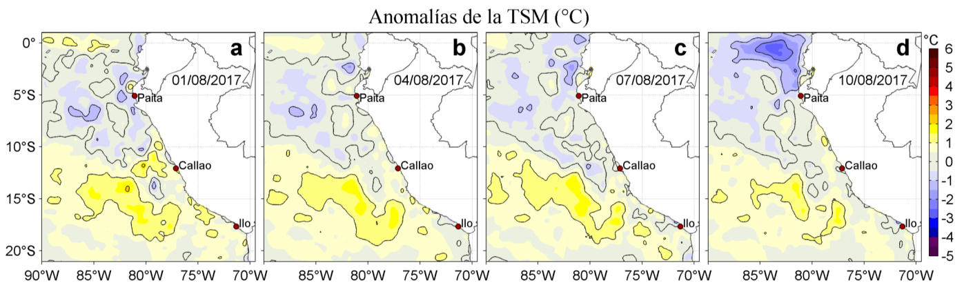
Figura 3. Anomalías de la Temperatura Superficial del Mar (°C) para los días: a) 01, b) 04, c) 07, y d) 10 de agosto de 2017. Las anomalías se calcularon respecto de la climatología para el periodo 2007-2016. Datos: OSTIA-UKMO-L4-GLOB-v2.0 (UK Met Office, 2012; Donlon et al, 2012). Procesamiento: LHF/AFIOF/DGIOCC/IMARPE.
