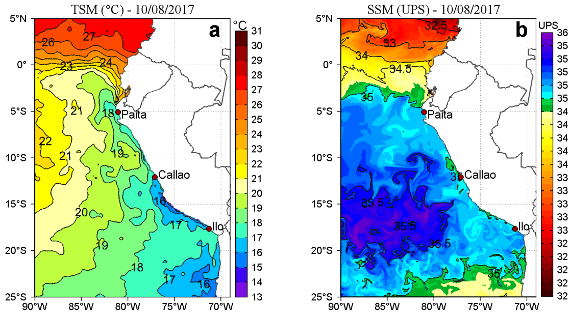
Figura 2. a) Temperatura superficial del mar (°C) y b) Salinidad superficial del mar (UPS) para el 10 de agosto respectivamente. Datos: OSTIA-UKMO-L4-GLOB-v2.0 (UK Met Office, 2012; Donlon et al, 2012) disponible en https://podaac.jpl.nasa.gov/dataset/OSTIA-UKMO-L4-GLOB-v2.0 para (a) y Hybrid Coordinate Ocean Model (HYCOM; Halliwell et al., 1998; 2000; Bleck, 2001) para (b). Procesamiento: LHF/AFIOF/DGIOCC/IMARPE.
