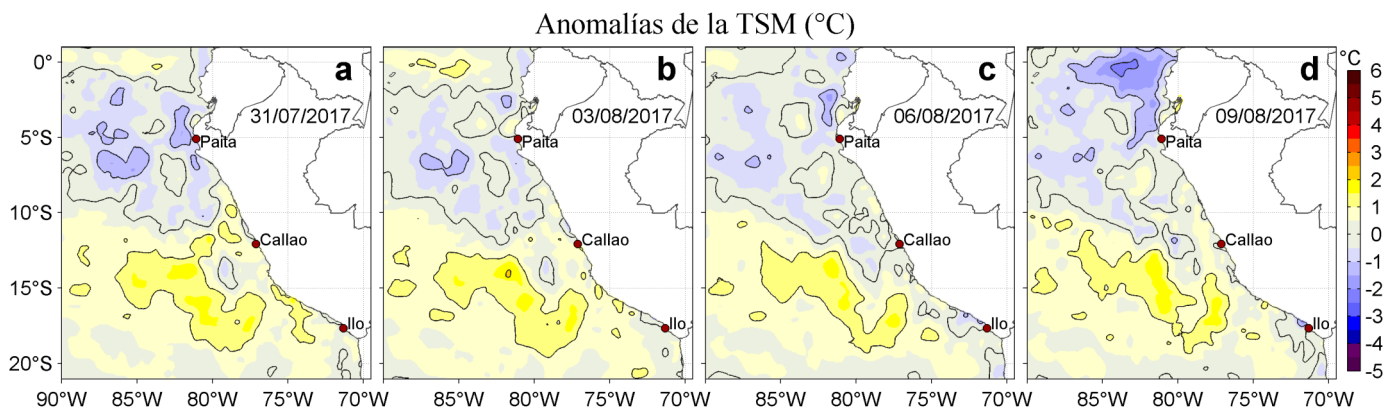
Figura 3. Anomalías de la Temperatura Superficial del Mar ( ^{\circ}\text{C} ) para los días: a) 31 de julio, b) 03, c) 06, y d) 09 de agosto de 2017. Las anomalías se calcularon respecto de la climatología para el periodo 2007-2016. Datos: OSTIA-UKMO-L4-GLOB-v2.0 (UK Met Office, 2012; Donlon et al, 2012). Procesamiento: LHF/AFIOF/DGIOCC/IMARPE.
