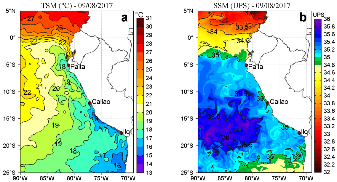
Figura 2. a) Temperatura superficial del mar ( ^{\circ}\text{C} ) y b) Salinidad superficial del mar (UPS) para el 09 de agosto respectivamente. Datos: OSTIA-UKMO-L4-GLOB-v2.0 (UK Met Office, 2012; Donlon et al, 2012) disponible en https://podaac.jpl.nasa.gov/dataset/OSTIA-UKMO-L4-GLOB-v2.0 para (a) y Hybrid Coordinate Ocean Model (HYCOM; Halliwell et al., 1998; 2000; Bleck, 2001) para (b). Procesamiento: LHF/AFIOF/DGIOCC/IMARPE.
