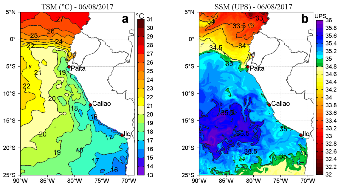
Figura 2. a) Temperatura superficial del mar ( ^{\circ}\text{C} ) y b) Salinidad superficial del mar (UPS) para el 06 de agosto. Datos: OSTIA-UKMO-L4-GLOB-v2.0 (UK Met Office, 2012; Donlon et al, 2012) disponible en https://podaac.jpl.nasa.gov/dataset/OSTIA-UKMO-L4-GLOB-v2.0 para (a) y Hybrid Coordinate Ocean Model (HYCOM; Halliwell et al., 1998; 2000; Bleck, 2001) para (b). Procesamiento: LHF/AFIOF/DGIOCC/IMARPE.
