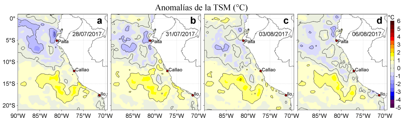
Figura 3. Anomalías de la Temperatura Superficial del Mar ( ^{\circ}\text{C} ) para los días: a) 28, y b) 31 de julio, y c) 03, y d) 06 de agosto de 2017. Las anomalías se calcularon respecto de la climatología para el periodo 2007-2016. Datos: OSTIA-UKMO-L4-GLOB-v2.0 (UK Met Office, 2012; Donlon et al, 2012). Procesamiento: LHF/AFIOF/DGIOCC/IMARPE.
