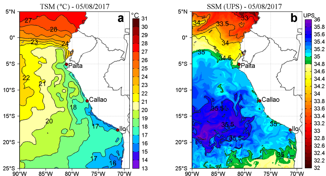
Figura 2. a) Temperatura superficial del mar ( ^{\circ}\text{C} ) y b) Salinidad superficial del mar (UPS) para el 05 de agosto. Datos: OSTIA-UKMO-L4-GLOB-v2.0 (UK Met Office, 2012; Donlon et al, 2012) disponible en https://podaac.jpl.nasa.gov/dataset/OSTIA-UKMO-L4-GLOB-v2.0 para (a) y Hybrid Coordinate Ocean Model (HYCOM; Halliwell et al., 1998; 2000; Bleck, 2001) para (b). Procesamiento: LHF/AFIOF/DGIOCC/IMARPE.
