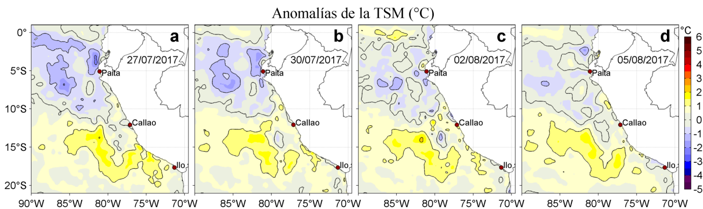
Figura 3. Anomalías de la Temperatura Superficial del Mar ( ^{\circ}\text{C} ) para los días: a) 27, b) 30 de julio, y c) 02, d) 05 de agosto de 2017. Las anomalías se calcularon respecto de la climatología para el periodo 2007-2016. Datos: OSTIA-UKMO-L4-GLOB-v2.0 (UK Met Office, 2012; Donlon et al, 2012). Procesamiento: LHF/AFIOF/DGIOCC/IMARPE.
