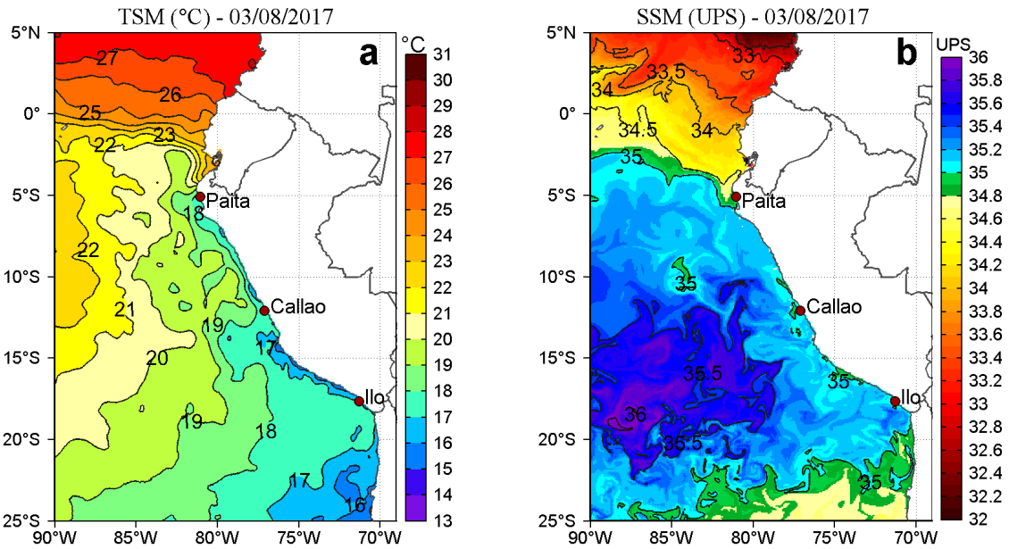
Figura 2. a) Temperatura superficial del mar (°C) y b) Salinidad superficial del mar (UPS) para el 03 de agosto. Datos: OSTIA-UKMO-L4-GLOB-v2.0 (UK Met Office, 2012; Donlon et al, 2012) disponible en https://podaac.jpl.nasa.gov/dataset/OSTIA-UKMO-L4-GLOB-v2.0 para (a) y Hybrid Coordinate Ocean Model (HYCOM; Halliwell et al., 1998; 2000; Bleck, 2001) para (b). Procesamiento: LHF/AFIOF/DGIOCC/IMARPE.
