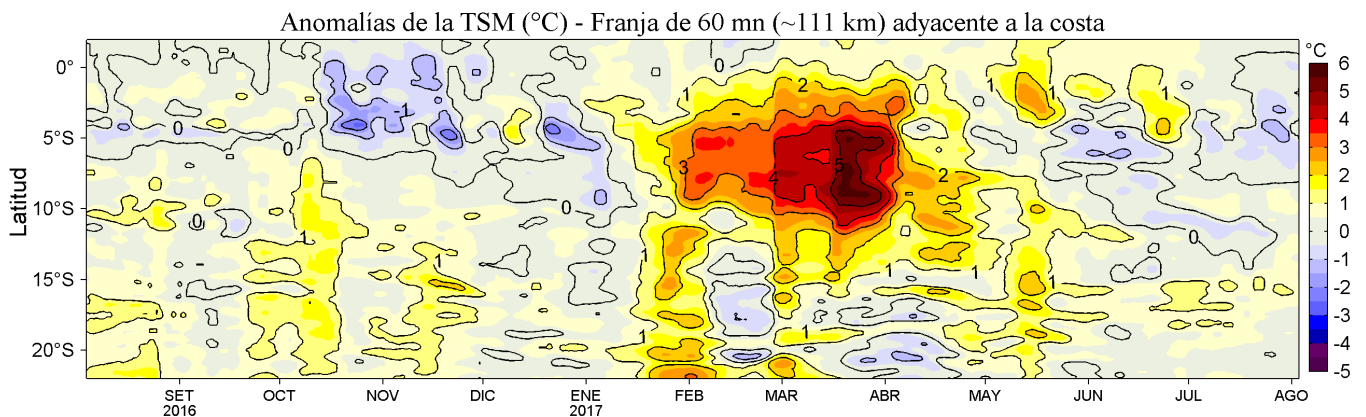
Figura 4. Variación promedio de las anomalías de la temperatura superficial del mar (°C) para una franja de 60 mn (~111 km) adyacente al litoral peruano para los últimos doce meses al 03 de agosto de 2017. Se distingue el calentamiento ocurrido de mediados de enero a fines de mayo de 2017 asociado con la presencia de El Niño Costero, evento que tuvo mayor impacto en la TSM (+5°C) en la segunda quincena de marzo. Datos: OSTIA-UKMO-L4-GLOB-v2.0 (UK Met. Office, 2012; Donlon et al, 2012) disponible en https://podaac.jpl.nasa.gov/dataset/OSTIA-UKMO-L4-GLOB-v2.0 . Las anomalías se calcularon con respecto al periodo 2007-2016. Procesamiento: LHF/AFIOF/DGIOCC/IMARPE.
