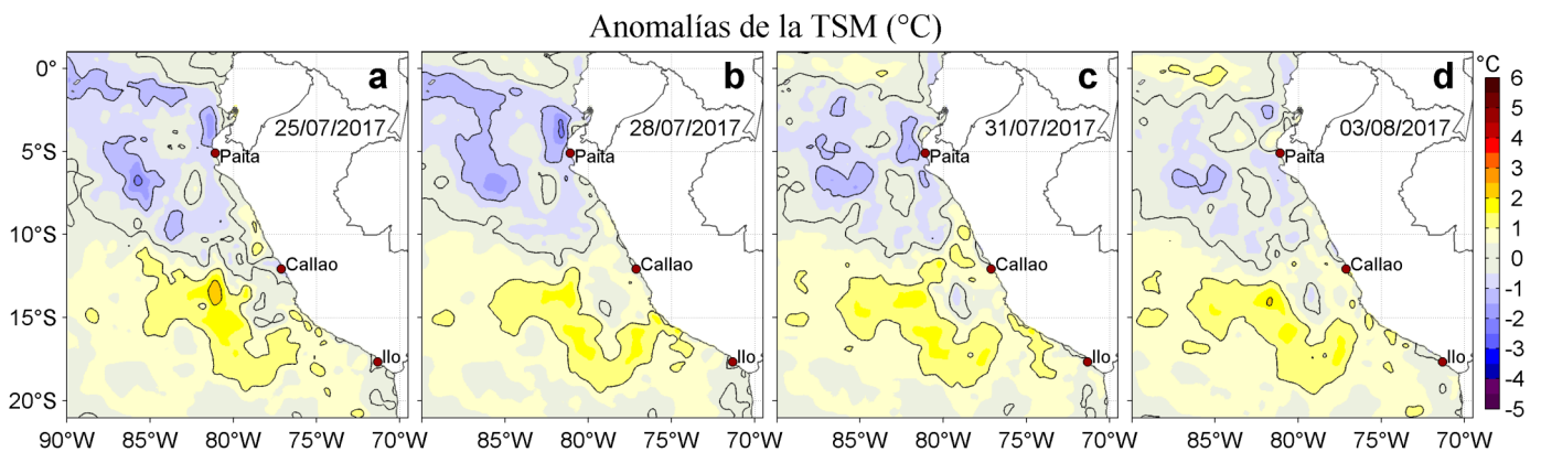
Figura 3. Anomalías de la Temperatura Superficial del Mar (°C) para los días: a) 25, b) 28, c) 31 de julio , y d) 03 de agosto de 2017. Las anomalías se calcularon respecto de la climatología para el periodo 2007-2016. Datos: OSTIA-UKMO-L4-GLOB-v2.0 (UK Met Office, 2012; Donlon et al, 2012). Procesamiento: LHF/AFIOF/DGIOCC/IMARPE.
