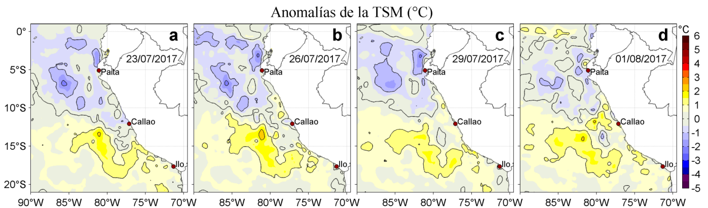
Figura 3. Anomalías de la Temperatura Superficial del Mar ( ^{\circ}\text{C} ) para los días: a) 23, b) 26, c) 29 de julio, y d) 01 de agosto de 2017. Las anomalías se calcularon respecto de la climatología para el periodo 2007-2016. Datos: OSTIA-UKMO-L4-GLOB-v2.0 (UK Met Office, 2012; Donlon et al, 2012). Procesamiento: LHF/AFIOF/DGIOCC/IMARPE.
