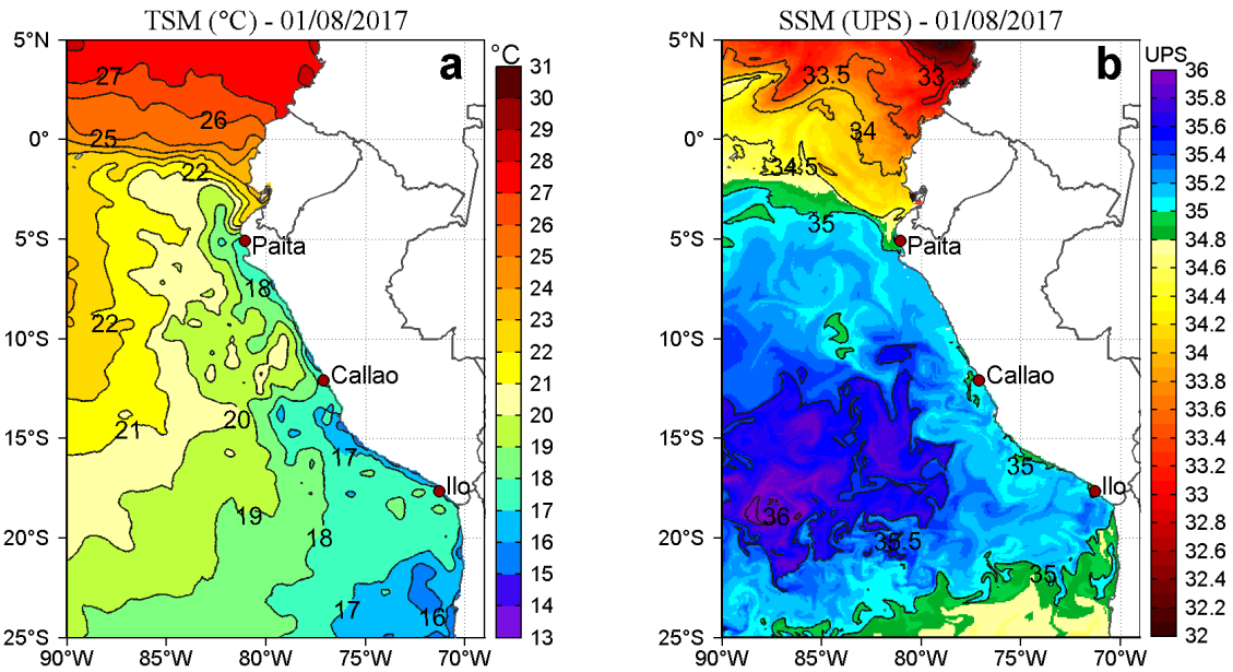
Figura 2. a) Temperatura superficial del mar ( ^{\circ}\text{C} ) y b) Salinidad superficial del mar (UPS) para el 01 de agosto. Datos: OSTIA-UKMO-L4-GLOB-v2.0 (UK Met Office, 2012; Donlon et al, 2012) disponible en https://podaac.jpl.nasa.gov/dataset/OSTIA-UKMO-L4-GLOB-v2.0 para (a) y Hybrid Coordinate Ocean Model (HYCOM; Halliwell et al., 1998; 2000; Bleck, 2001) para (b). Procesamiento: LHF/AFIOF/DGIOCC/IMARPE.
