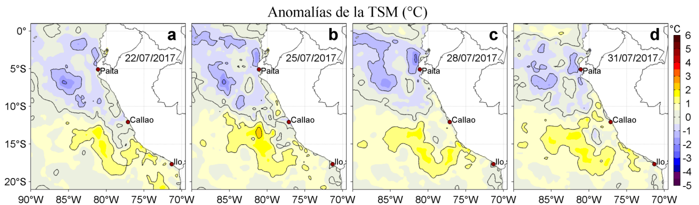
Figura 3. Anomalías de la Temperatura Superficial del Mar ( ^{\circ}\text{C} ) para los días: a) 22, b) 25, c) 28, y d) 31 de julio de 2017. Las anomalías se calcularon respecto de la climatología para el periodo 2007-2016. Datos: OSTIA-UKMO-L4-GLOB-v2.0 (UK Met Office, 2012; Donlon et al, 2012). Procesamiento: LHF/AFIOF/DGIOCC/IMARPE.
