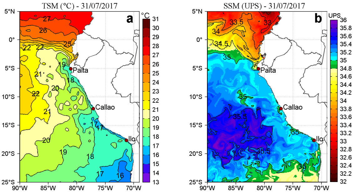
Figura 2. a) Temperatura superficial del mar ( ^{\circ}\text{C} ) y b) Salinidad superficial del mar (UPS) para el 31 de julio. Datos: OSTIA-UKMO-L4-GLOB-v2.0 (UK Met Office, 2012; Donlon et al, 2012) disponible en https://podaac.jpl.nasa.gov/dataset/OSTIA-UKMO-L4-GLOB-v2.0 para (a) y Hybrid Coordinate Ocean Model (HYCOM; Halliwell et al., 1998; 2000; Bleck, 2001) para (b). Procesamiento: LHF/AFIOF/DGIOCC/IMARPE.
