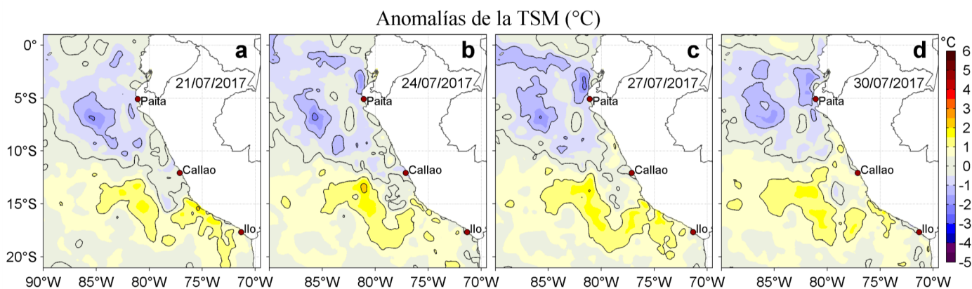
Figura 3. Anomalías de la Temperatura Superficial del Mar ( ^{\circ}\text{C} ) para los días: a) 21, b) 24, c) 27, y d) 30 de julio de 2017. Las anomalías se calcularon respecto de la climatología para el periodo 2007-2016. Datos: OSTIA-UKMO-L4-GLOB-v2.0 (UK Met Office, 2012; Donlon et al, 2012). Procesamiento: LHF/AFIOF/DGIOCC/IMARPE.
