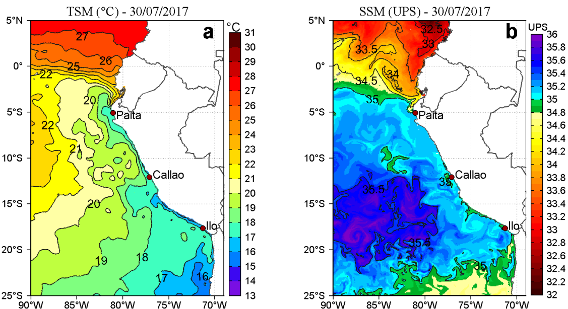
Figura 2. a) Temperatura superficial del mar ( ^{\circ}\text{C} ) y b) Salinidad superficial del mar (UPS) para el 30 de julio respectivamente. Datos: OSTIA-UKMO-L4-GLOB-v2.0 (UK Met Office, 2012; Donlon et al, 2012) disponible en https://podaac.jpl.nasa.gov/dataset/OSTIA-UKMO-L4-GLOB-v2.0 para (a) y Hybrid Coordinate Ocean Model (HYCOM; Halliwell et al., 1998; 2000; Bleck, 2001) para (b). Procesamiento: LHF/AFIOF/DGIOCC/IMARPE.
