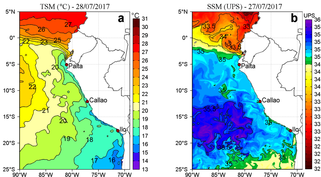
Figura 2. a) Temperatura superficial del mar ( ^{\circ}\text{C} ) y b) Salinidad superficial del mar (UPS) para el 28 y 27 de julio respectivamente. Datos: OSTIA-UKMO-L4-GLOB-v2.0 (UK Met Office, 2012; Donlon et al, 2012) disponible en https://podaac.jpl.nasa.gov/dataset/OSTIA-UKMO-L4-GLOB-v2.0 para (a) y Hybrid Coordinate Ocean Model (HYCOM; Halliwell et al., 1998; 2000; Bleck, 2001) para (b). Procesamiento: LHF/AFIOF/DGIOCC/IMARPE.
