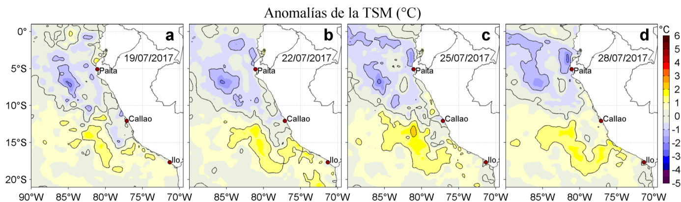
Figura 3. Anomalías de la Temperatura Superficial del Mar ( ^{\circ}\text{C} ) para los días: a) 19, b) 22, c) 25, y d) 28 de julio de 2017. Las anomalías se calcularon respecto de la climatología para el periodo 2007-2016. Datos: OSTIA-UKMO-L4-GLOB-v2.0 (UK Met Office, 2012; Donlon et al, 2012). Procesamiento: LHF/AFIOF/DGIOCC/IMARPE.
