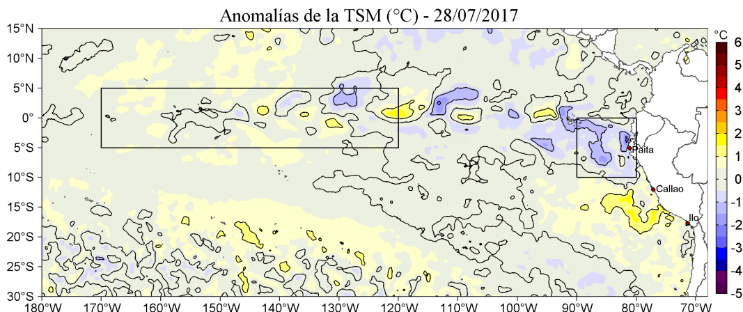
Figura 1. Anomalías de la temperatura superficial del mar (°C) en el océano Pacífico tropical. Las regiones Niño 3.4 (5°N - 5°S, 170°W - 120°W) y Niño 1+2 (0° - 10°S, 90°W—80°W) en los sectores central y oriental del océano, respectivamente, están delimitadas con una línea de color negro. Climatología: 2007-2016. Datos: OSTIA-UKMO-L4-GLOB-v2.0 (UK Met Office, 2012; Donlon et al, 2012) disponible en https://podaac.jpl.nasa.gov/dataset/OSTIA-UKMO-L4-GLOB-v2.0 . Procesamiento: IMARPE.
