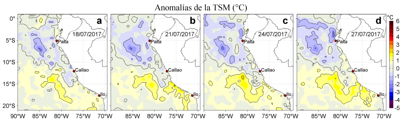
Figura 3. Anomalías de la Temperatura Superficial del Mar (°C) para los días: a) 18, b) 21, c) 24, y d) 27 de julio de 2017. Las anomalías se calcularon respecto de la climatología para el periodo 2007-2016. Datos: OSTIA-UKMO-L4-GLOB-v2.0 (UK Met Office, 2012; Donlon et al, 2012). Procesamiento: LHF/AFIOF/DGIOCC/IMARPE.
