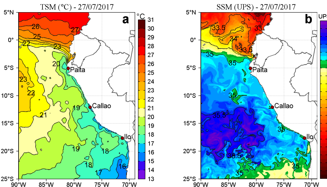
Figura 2. a) Temperatura superficial del mar (°C) y b) Salinidad superficial del mar (UPS) para el 27 de julio. Datos: OSTIA-UKMO-L4-GLOB-v2.0 (UK Met Office, 2012; Donlon et al, 2012) disponible en https://podaac.jpl.nasa.gov/dataset/OSTIA-UKMO-L4-GLOB-v2.0 ) para (a) y Hybrid Coordinate Ocean Model (HYCOM; Halliwell et al., 1998; 2000; Bleck, 2001) para (b). Procesamiento: LHF/AFIOF/DGIOCC/IMARPE.
