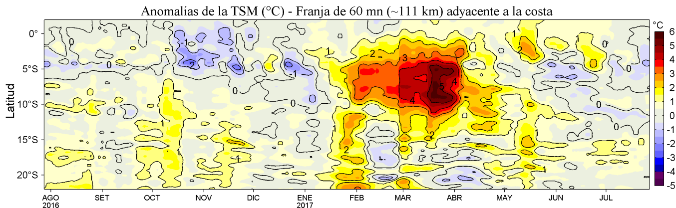
Figura 4. Variación promedio de las anomalías de la temperatura superficial del mar (°C) para una franja de 60 mn (~111 km) adyacente al litoral peruano para los últimos doce meses al 27 de julio de 2017. Se distingue el calentamiento ocurrido de mediados de enero a fines de mayo de 2017 asociado con la presencia de El Niño Costero, evento que tuvo mayor impacto en la TSM (+5°C) en la segunda quincena de marzo. Datos: OSTIA-UKMO-L4-GLOB-v2.0 (UK Met. Office, 2012; Donlon et al, 2012) disponible en https://podaac.jpl.nasa.gov/dataset/OSTIA-UKMO-L4-GLOB-v2.0 ). Las anomalías se calcularon con respecto al periodo 2007-2016. Procesamiento: LHF/AFIOF/DGIOCC/IMARPE.
