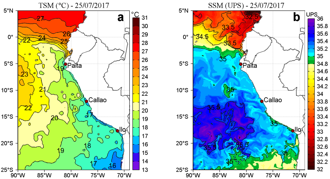
Figura 2. a) Temperatura superficial del mar ( ^{\circ}\text{C} ) y b) Salinidad superficial del mar (UPS) para el 25 de julio. Datos: OSTIA-UKMO-L4-GLOB-v2.0 (UK Met Office, 2012; Donlon et al, 2012) disponible en https://podaac.jpl.nasa.gov/dataset/OSTIA-UKMO-L4-GLOB-v2.0 para (a) y Hybrid Coordinate Ocean Model (HYCOM; Halliwell et al., 1998; 2000; Bleck, 2001) para (b). Procesamiento: LHF/AFIOF/DGIOCC/IMARPE.
