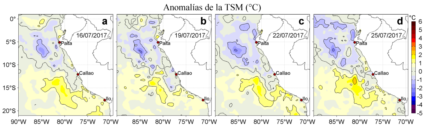
Figura 3. Anomalías de la Temperatura Superficial del Mar ( ^{\circ}\text{C} ) para los días: a) 16, b) 19, c) 22, y d) 25 de julio de 2017. Las anomalías se calcularon respecto de la climatología para el periodo 2007-2016. Datos: OSTIA-UKMO-L4-GLOB-v2.0 (UK Met Office, 2012; Donlon et al, 2012). Procesamiento: LHF/AFIOF/DGIOCC/IMARPE.
