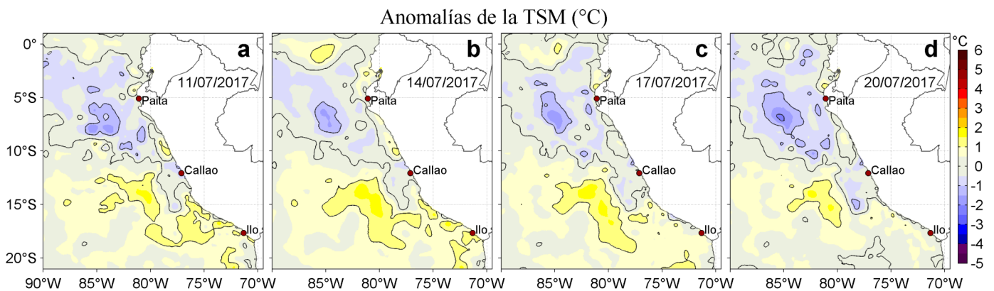
Figura 3. Anomalías de la Temperatura Superficial del Mar (°C) para los días: a) 11, b) 14, c) 17, y d) 20 de julio de 2017. Las anomalías se calcularon respecto de la climatología para el periodo 2007-2016. Datos: OSTIA-UKMO-L4-GLOB-v2.0 (UK Met Office, 2012; Donlon et al, 2012). Procesamiento: LHF/AFIOF/DGIOCC/IMARPE.
