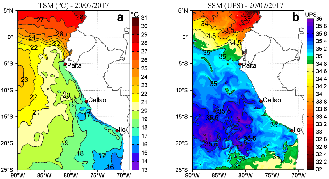
Figura 2. a) Temperatura superficial del mar (°C) y b) Salinidad superficial del mar (UPS) para el 20 de julio. Datos: OSTIA-UKMO-L4-GLOB-v2.0 (UK Met Office, 2012; Donlon et al, 2012) disponible en https://podaac.jpl.nasa.gov/dataset/OSTIA-UKMO-L4-GLOB-v2.0 para (a) y Hybrid Coordinate Ocean Model (HYCOM; Halliwell et al., 1998; 2000; Bleck, 2001) para (b). Procesamiento: LHF/AFIOF/DGIOCC/IMARPE.
