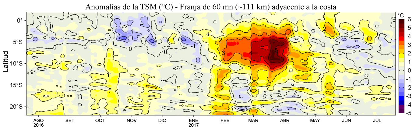
Figura 4. Variación promedio de las anomalías de la temperatura superficial del mar (°C) para una franja de 60 mn (~111 km) adyacente al litoral peruano para los últimos doce meses al 19 de julio de 2017. Se distingue el calentamiento ocurrido de mediados de enero a fines de mayo de 2017 asociado con la presencia de El Niño Costero, evento que tuvo mayor impacto en la TSM (+5°C) en la segunda quincena de marzo. Datos: OSTIA-UKMO-L4-GLOB-v2.0 (UK Met Office, 2012; Donlon et al, 2012) disponible en https://podaac.jpl.nasa.gov/dataset/OSTIA-UKMO-L4-GLOB-v2.0 . Las anomalías se calcularon con respecto al periodo 2007-2016. Procesamiento: LHF/AFIOF/DGIOCC/IMARPE.
