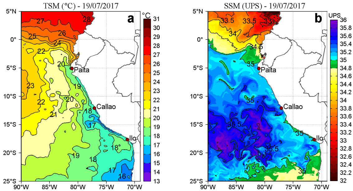
Figura 2. a) Temperatura superficial del mar (°C) y b) Salinidad superficial del mar (UPS) para el 19 de julio. Datos: OSTIA-UKMO-L4-GLOB-v2.0 (UK Met Office, 2012; Donlon et al, 2012) disponible en https://podaac.jpl.nasa.gov/dataset/OSTIA-UKMO-L4-GLOB-v2.0 para (a) y Hybrid Coordinate Ocean Model (HYCOM; Halliwell et al., 1998; 2000; Bleck, 2001) para (b). Procesamiento: LHF/AFIOF/DGIOCC/IMARPE.
