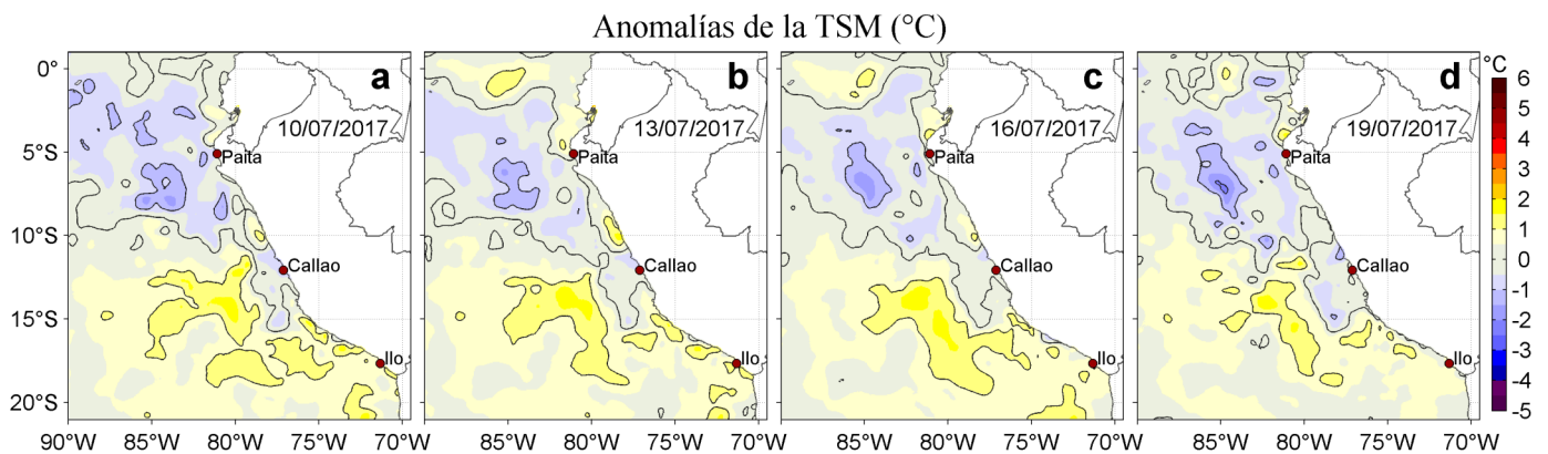
Figura 3. Anomalías de la Temperatura Superficial del Mar (°C) para los días: a) 10, b) 13, c) 16, y d) 19 de julio de 2017. Las anomalías se calcularon respecto de la climatología para el periodo 2007-2016. Datos: OSTIA-UKMO-L4-GLOB-v2.0 (UK Met Office, 2012; Donlon et al, 2012). Procesamiento: LHF/AFIOF/DGIOCC/IMARPE.
