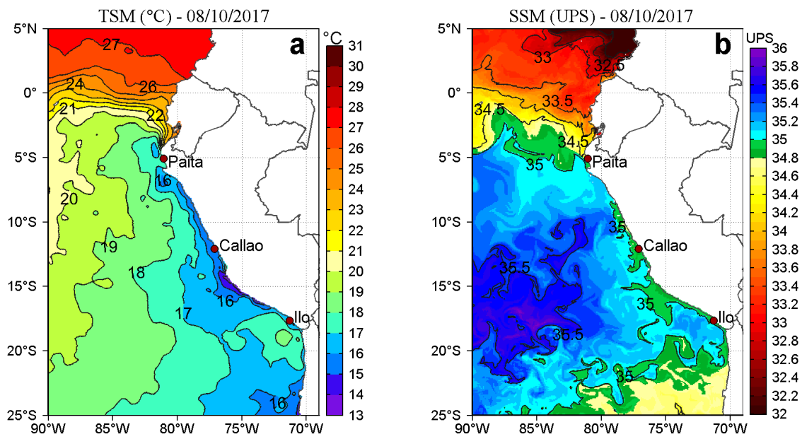
Figura 2. a) Temperatura superficial del mar ( ^{\circ}\text{C} ) y b) Salinidad superficial del mar (UPS) para el 08 de octubre. Datos: OSTIA-UKMO-L4-GLOB-v2.0 (UK Met Office, 2012; Donlon et al, 2012) disponible en https://podaac.jpl.nasa.gov/dataset/OSTIA-UKMO-L4-GLOB-v2.0 para (a) y Hybrid Coordinate Ocean Model (HYCOM; Halliwell et al., 1998; 2000; Bleck, 2001) para (b). Procesamiento: LHF/AFIOF/DGIOCC/IMARPE.
