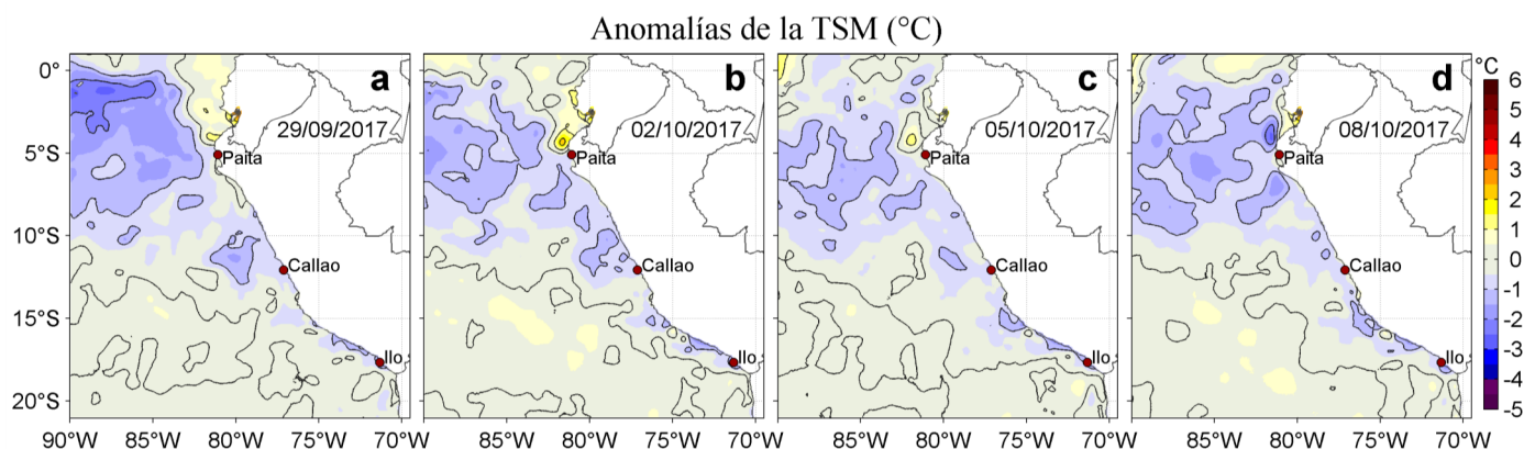
Figura 3. Anomalías de la Temperatura Superficial del Mar ( ^{\circ}\text{C} ) para los días: a) 29 de setiembre, b) 02, c) 05, y d) 08 de octubre de 2017. Las anomalías se calcularon respecto de la climatología para el periodo 2007-2016. Datos: OSTIA-UKMO-L4-GLOB-v2.0 (UK Met Office, 2012; Donlon et al, 2012). Procesamiento: LHF/AFIOF/DGIOCC/IMARPE.
