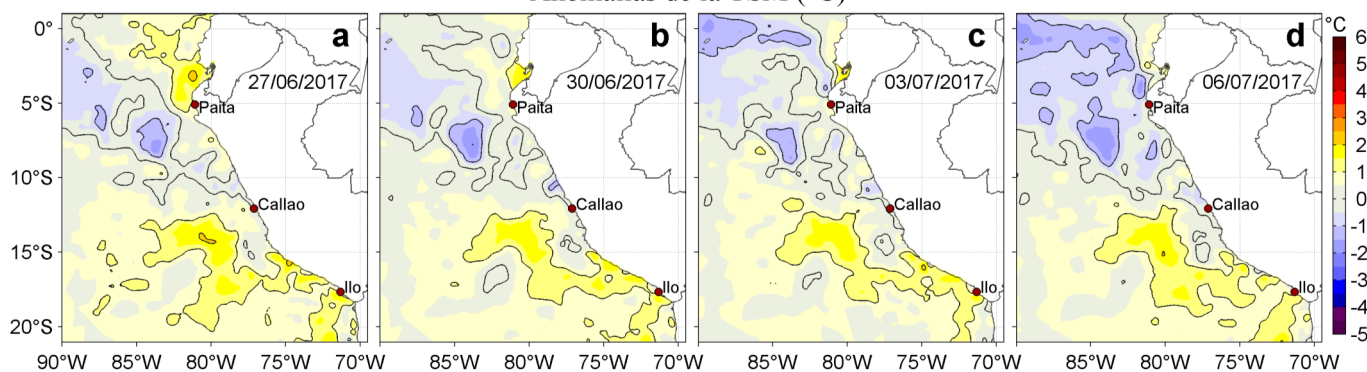
Figura 3. Anomalías de la Temperatura Superficial del Mar ( ^{\circ}\text{C} ) para los días: a) 27 y b) 30 de junio, c) 03, y d) 06 de julio de 2017. Las anomalías se calcularon respecto de la climatología para el periodo 2007-2016. Datos: OSTIA-UKMO-L4-GLOB-v2.0 (UK Met Office, 2012; Donlon et al, 2012). Procesamiento: LHF/AFIOF/DGIOCC/IMARPE.
