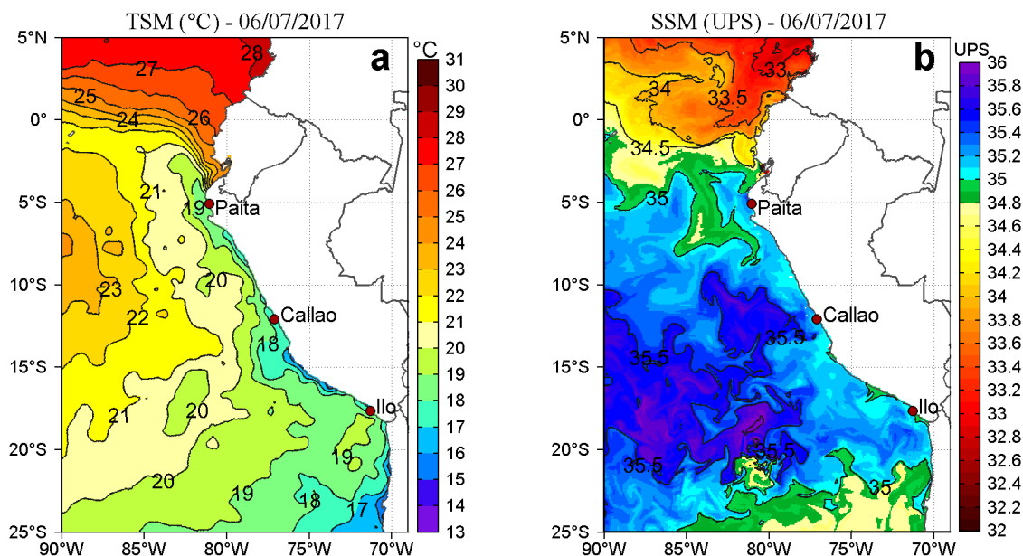
Figura 2. a) Temperatura superficial del mar ( ^{\circ}\text{C} ) y b) Salinidad superficial del mar (UPS) para el 06 de julio. Datos: OSTIA-UKMO-L4-GLOB-v2.0 (UK Met Office, 2012; Donlon et al, 2012) disponible en https://podaac.jpl.nasa.gov/dataset/OSTIA-UKMO-L4-GLOB-v2.0 para (a) y Hybrid Coordinate Ocean Model (HYCOM; Halliwell et al., 1998; 2000; Bleck, 2001) para (b). Procesamiento: AFSR/DGIHSA/IMARPE.
