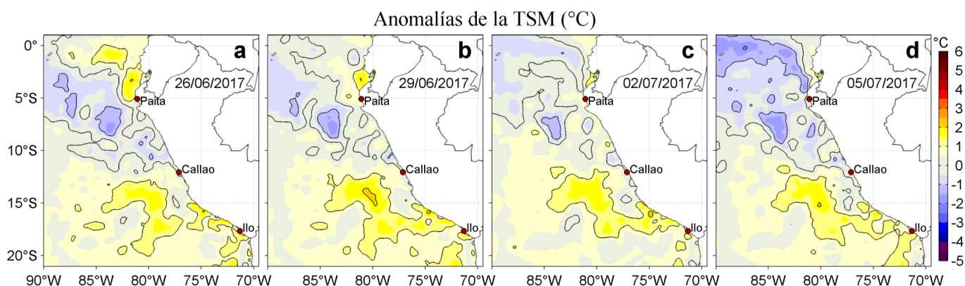
Figura 3. Anomalías de la Temperatura Superficial del Mar (°C) para los días: a) 26, b) 29 de junio, y c) 02, d) 05 de julio de 2017. Las anomalías se calcularon respecto de la climatología para el periodo 2007-2016. Datos: OSTIA-UKMO-L4-GLOB-v2.0 (UK Met Office, 2012; Donlon et al, 2012). Procesamiento: LHF/AFIOF/DGIOCC/IMARPE.
