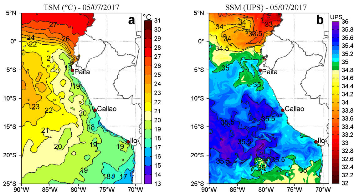
Figura 2. a) Temperatura superficial del mar (°C) y b) Salinidad superficial del mar (UPS) para el 05 de julio. Datos: OSTIA-UKMO-L4-GLOB-v2.0 (UK Met Office, 2012; Donlon et al, 2012) disponible en https://podaac.jpl.nasa.gov/dataset/OSTIA-UKMO-L4-GLOB-v2.0 para (a) y Hybrid Coordinate Ocean Model (HYCOM; Halliwell et al., 1998; 2000; Bleck, 2001) para (b). Procesamiento: AFSR/DGIHSA/IMARPE.
