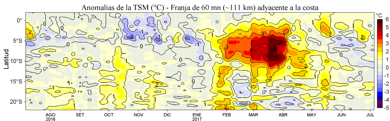
Figura 4. Variación promedio de las anomalías de la temperatura superficial del mar (°C) para una franja de 60 mn (~111 km) adyacente al litoral peruano para los últimos doce meses al 05 de julio de 2017. Se distingue el calentamiento ocurrido de mediados de enero a fines de mayo de 2017 asociado con la presencia de El Niño Costero, evento que tuvo mayor impacto en la TSM (+5°C) en la segunda quincena de marzo. Datos: OSTIA-UKMO-L4-GLOB-v2.0 (UK Met Office, 2012; Donlon et al, 2012) disponible en https://podaac.jpl.nasa.gov/dataset/OSTIA-UKMO-L4-GLOB-v2.0 ). Las anomalías se calcularon con respecto al periodo 2007-2016. Procesamiento: LHF/AFIOF/DGIOCC/IMARPE.
