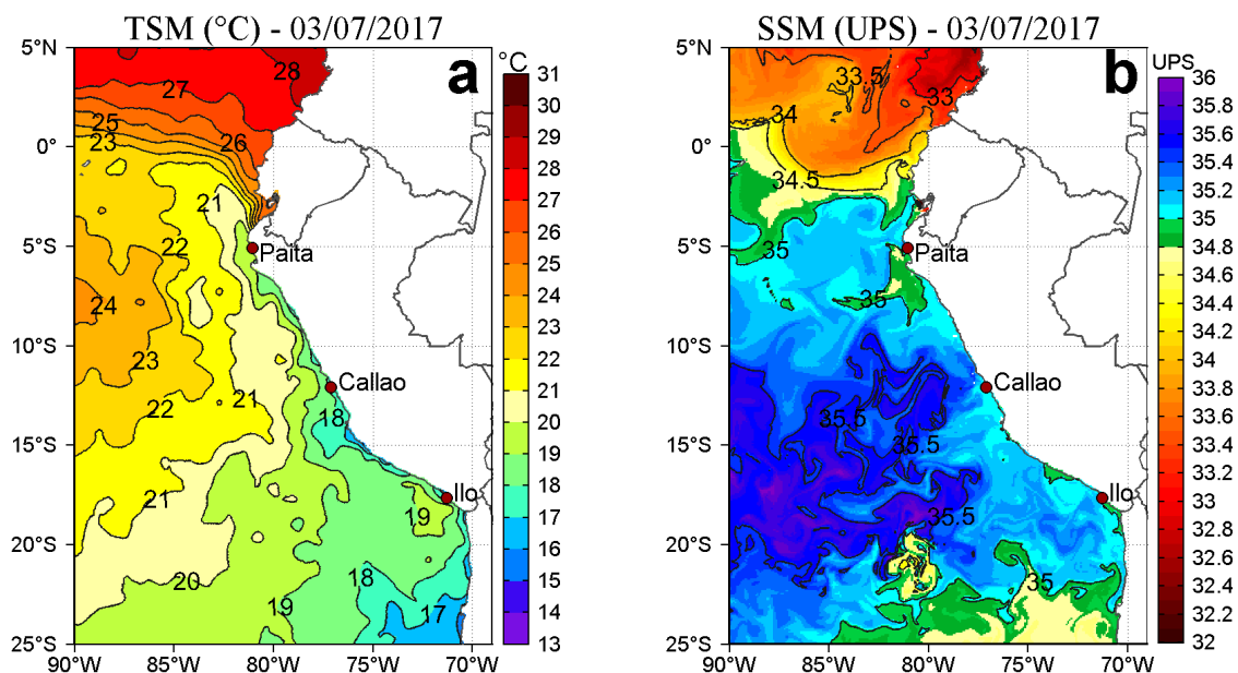
Figura 2. a) Temperatura superficial del mar (°C) y b) Salinidad superficial del mar (UPS) para el 03 de julio. Datos: OSTIA-UKMO-L4-GLOB-v2.0 (UK Met Office, 2012; Donlon et al, 2012) disponible en https://podaac.jpl.nasa.gov/dataset/OSTIA-UKMO-L4-GLOB-v2.0 para (a) y Hybrid Coordinate Ocean Model (HYCOM; Halliwell et al., 1998; 2000; Bleck, 2001) para (b). Procesamiento: AFSR/DGIHSA/IMARPE.
