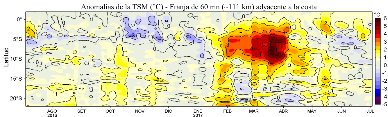
Figura 4. Variación promedio de las anomalías de la temperatura superficial del mar (°C) para una franja de 60 mn (~111 km) adyacente al litoral peruano para los últimos doce meses al 03 de julio de 2017. Se distingue el calentamiento ocurrido de mediados de enero a fines de mayo de 2017 asociado con la presencia de El Niño Costero, evento que tuvo mayor impacto en la TSM (+5°C) en la segunda quincena de marzo. Datos: OSTIA-UKMO-L4-GLOB-v2.0 (UK Met Office, 2012; Donlon et al, 2012) disponible en https://podaac.jpl.nasa.gov/dataset/OSTIA-UKMO-L4-GLOB-v2.0 . Las anomalías se calcularon con respecto al periodo 2007-2016. Procesamiento: LHF/AFIOF/DGIOCC/IMARPE.
