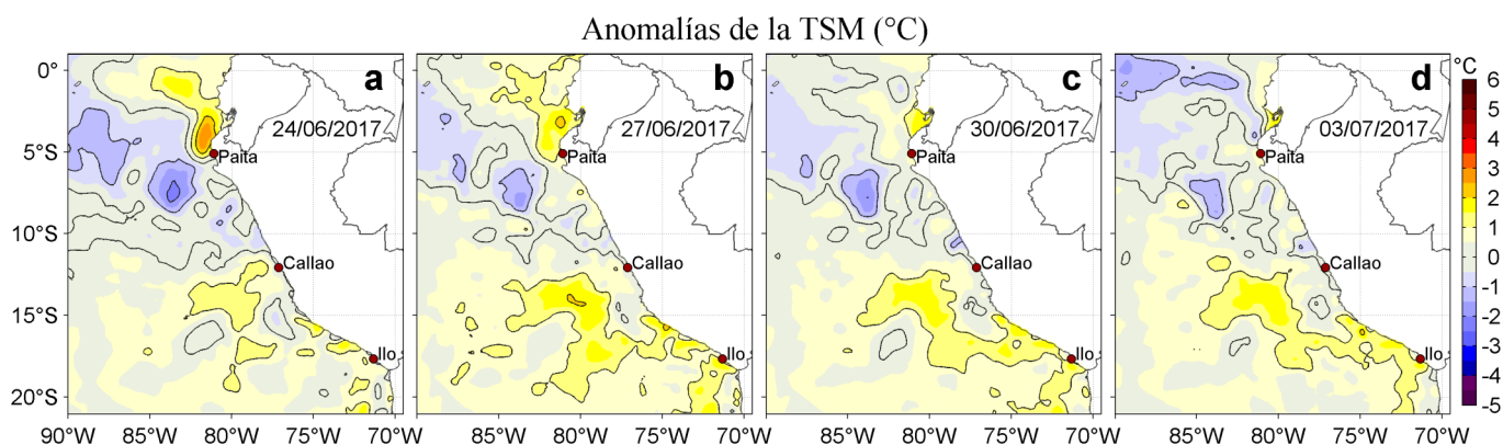
Figura 3. Anomalías de la Temperatura Superficial del Mar (°C) para los días: a) 24, b) 27, c) 30, de junio, y d) 03 de julio de 2017. Las anomalías se calcularon respecto de la climatología para el periodo 2007-2016. Datos: OSTIA-UKMO-L4-GLOB-v2.0 (UK Met Office, 2012; Donlon et al, 2012). Procesamiento: LHF/AFIOF/DGIOCC/IMARPE.
