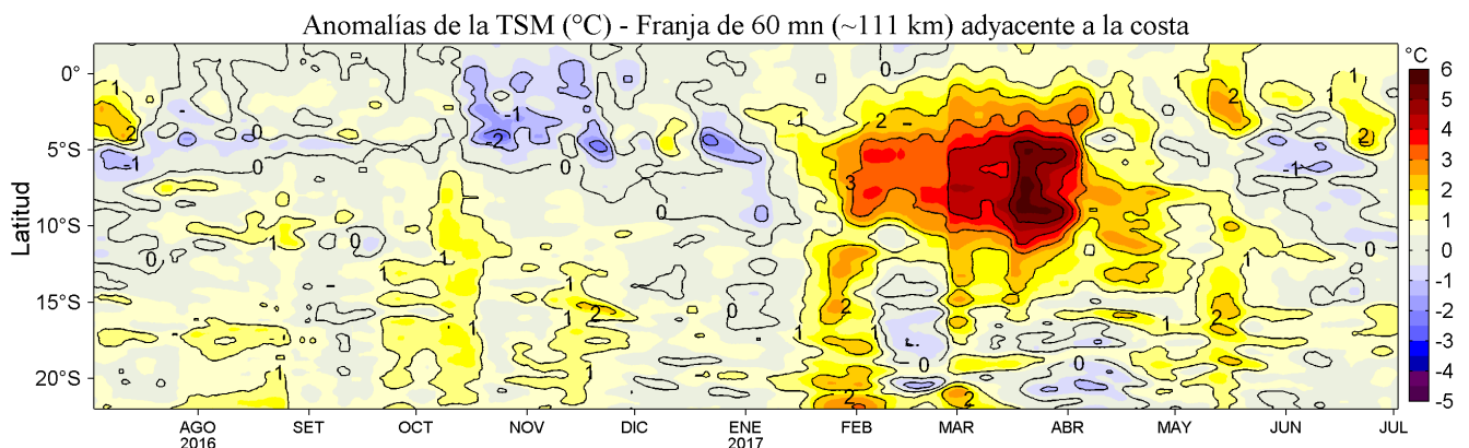
Figura 4. Variación promedio de las anomalías de la temperatura superficial del mar (°C) para una franja de 60 mn (~111 km) adyacente al litoral peruano para los últimos doce meses al 02 de julio de 2017. Se distingue el calentamiento ocurrido de mediados de enero a fines de mayo de 2017 asociado con la presencia de El Niño Costero, evento que tuvo mayor impacto en la TSM (+5°C) en la segunda quincena de marzo. Datos: OSTIA-UKMO-L4-GLOB-v2.0 (UK Met Office, 2012; Donlon et al, 2012) disponible en https://podaac.jpl.nasa.gov/dataset/OSTIA-UKMO-L4-GLOB-v2.0 . Las anomalías se calcularon con respecto al periodo 2007-2016. Procesamiento: LHF/AFIOF/DGIOCC/IMARPE.
