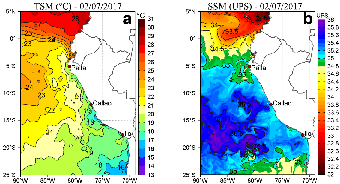
Figura 2. a) Temperatura superficial del mar (°C) y b) Salinidad superficial del mar (UPS) para el 02 de julio. Datos: OSTIA-UKMO-L4-GLOB-v2.0 (UK Met Office, 2012; Donlon et al, 2012) disponible en https://podaac.jpl.nasa.gov/dataset/OSTIA-UKMO-L4-GLOB-v2.0 para (a) y Hybrid Coordinate Ocean Model (HYCOM; Halliwell et al., 1998; 2000; Bleck, 2001) para (b). Procesamiento: AFSR/DGIHSA/IMARPE.
