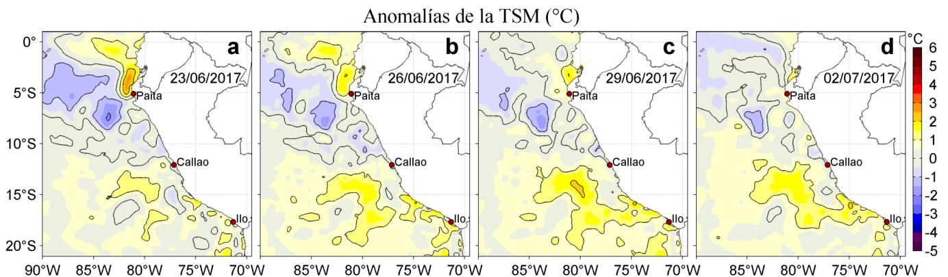
Figura 3. Anomalías de la Temperatura Superficial del Mar (°C) para los días: a) 23, b) 26, c) 29, de junio, y d) 02 de julio de 2017. Las anomalías se calcularon respecto de la climatología para el periodo 2007-2016. Datos: OSTIA-UKMO-L4-GLOB-v2.0 (UK Met Office, 2012; Donlon et al, 2012). Procesamiento: LHF/AFIOF/DGIOCC/IMARPE.
