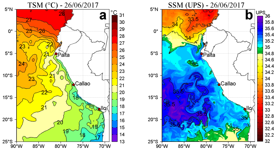
Figura 2. a) Temperatura superficial del mar ( ^{\circ}\text{C} ) y b) Salinidad superficial del mar (UPS) para el 26 de junio. Datos: OSTIA-UKMO-L4-GLOB-v2.0 (UK Met Office, 2012; Donlon et al, 2012) disponible en https://podaac.jpl.nasa.gov/dataset/OSTIA-UKMO-L4-GLOB-v2.0 para (a) y Hybrid Coordinate Ocean Model (HYCOM; Halliwell et al., 1998; 2000; Bleck, 2001) para (b). Procesamiento: AFSR/DGIHSA/IMARPE.
