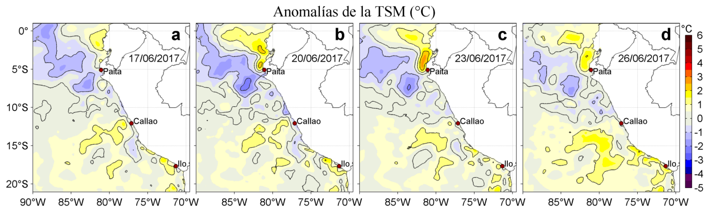
Figura 3. Anomalías de la Temperatura Superficial del Mar ( ^{\circ}\text{C} ) para los días: a) 17, b) 20, c) 23, y d) 26 de junio de 2017. Las anomalías se calcularon respecto de la climatología para el periodo 2007-2016. Datos: OSTIA-UKMO-L4-GLOB-v2.0 (UK Met Office, 2012; Donlon et al, 2012). Procesamiento: LHF/AFIOF/DGIOCC/IMARPE.
