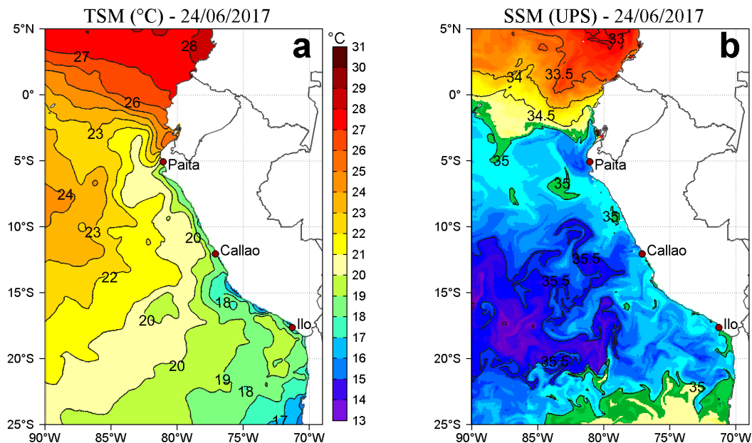
Figura 2. a) Temperatura superficial del mar ( ^{\circ}\text{C} ) y b) Salinidad superficial del mar (UPS) para el 24 de junio. Datos: OSTIA-UKMO-L4-GLOB-v2.0 (UK Met Office, 2012; Donlon et al, 2012) disponible en https://podaac.jpl.nasa.gov/dataset/OSTIA-UKMO-L4-GLOB-v2.0 para (a) y Hybrid Coordinate Ocean Model (HYCOM; Halliwell et al., 1998; 2000; Bleck, 2001) para (b). Procesamiento: AFSR/DGIHSA/IMARPE.
