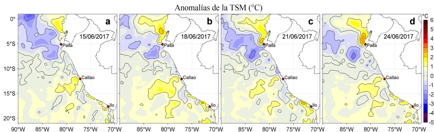
Figura 3. Anomalías de la Temperatura Superficial del Mar ( ^{\circ}\text{C} ) para los días: a) 15, b) 18, c) 21, y d) 24 de junio de 2017. Las anomalías se calcularon respecto de la climatología para el periodo 2007-2016. Datos: OSTIA-UKMO-L4-GLOB-v2.0 (UK Met Office, 2012; Donlon et al, 2012). Procesamiento: LHF/AFIOF/DGIOCC/IMARPE.
