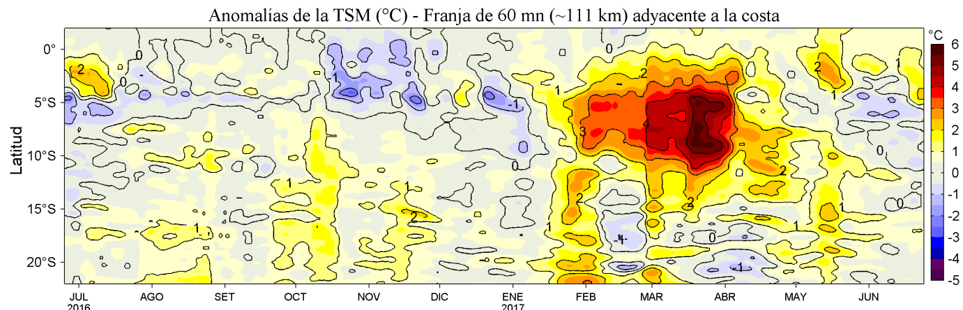
Figura 4. Variación promedio de las anomalías de la temperatura superficial del mar ( ^{\circ}\text{C} ) para una franja de 60 mn ( \sim 111 km) adyacente a la costa litoral peruano para los últimos doce meses al 24 de junio de 2017. Se distingue el calentamiento ocurrido de mediados de enero a fines de mayo de 2017 asociado con la presencia de El Niño Costero, evento que tuvo mayor impacto en la TSM ( +5^{\circ}\text{C} ) en la segunda quincena de marzo. Datos: OSTIA-UKMO-L4-GLOB-v2.0 (UK Met Office, 2012; Donlon et al, 2012) disponible en https://podaac.jpl.nasa.gov/dataset/OSTIA-UKMO-L4-GLOB-v2.0 . Las anomalías se calcularon con respecto al periodo 2007-2016. Procesamiento: LHF/AFIOF/DGIOCC/IMARPE.
