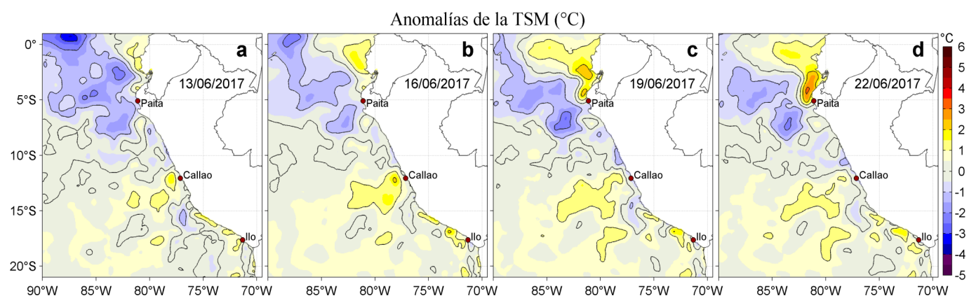
Figura 3. Anomalías de la Temperatura Superficial del Mar (°C) para los días: a) 13, b) 16, c) 19, y d) 22 de junio de 2017. Las anomalías se calcularon respecto de la climatología para el periodo 2007-2016. Datos: OSTIA-UKMO-L4-GLOB-v2.0 (UK Met Office, 2012; Donlon et al, 2012). Procesamiento: LHF/AFIOF/DGIOCC/IMARPE.
