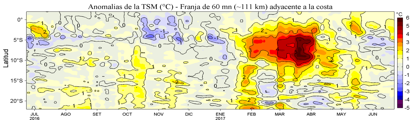
Figura 4. Variación promedio de las anomalías de la temperatura superficial del mar (°C) para una franja de 60 mn (~111 km) adyacente al litoral peruano para los últimos doce meses al 22 de junio de 2017. Se distingue el calentamiento ocurrido de mediados de enero a fines de mayo de 2017 asociado con la presencia de El Niño Costero, evento que tuvo mayor impacto en la TSM (+5°C) en la segunda quincena de marzo. Datos: OSTIA-UKMO-L4-GLOB-v2.0 (UK Met Office, 2012; Donlon et al, 2012) disponible en https://podaac.jpl.nasa.gov/dataset/OSTIA-UKMO-L4-GLOB-v2.0 ). Las anomalías se calcularon con respecto al periodo 2007-2016. Procesamiento: LHF/AFIOF/DGIOCC/IMARPE.
