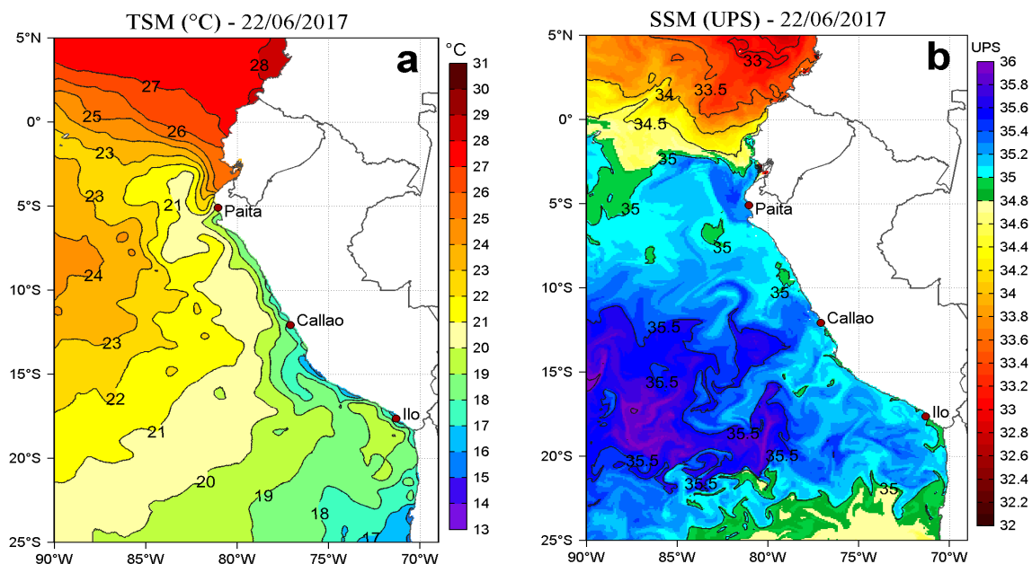
Figura 2. a) Temperatura superficial del mar (°C) y b) Salinidad superficial del mar (UPS) para el 22 de junio. Datos: OSTIA-UKMO-L4-GLOB-v2.0 (UK Met Office, 2012; Donlon et al, 2012) disponible en https://podaac.jpl.nasa.gov/dataset/OSTIA-UKMO-L4-GLOB-v2.0 ) para (a) y Hybrid Coordinate Ocean Model (HYCOM; Halliwell et al., 1998; 2000; Bleck, 2001) para (b). Procesamiento: LHF/AFIOF/DGIOCC/IMARPE.
