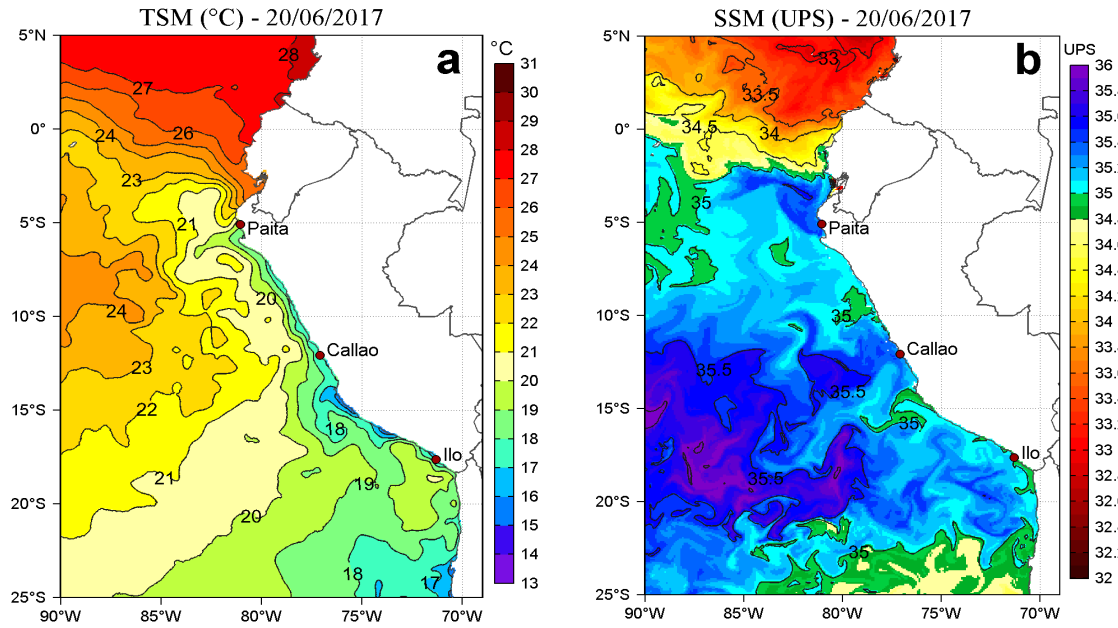
Figura 2. a) Temperatura superficial del mar ( ^{\circ}\text{C} ) y b) Salinidad superficial del mar (UPS) para el 20 de junio. Datos: OSTIA-UKMO-L4-GLOB-v2.0 (UK Met Office, 2012; Donlon et al, 2012) disponible en https://podaac.jpl.nasa.gov/dataset/OSTIA-UKMO-L4-GLOB-v2.0 para (a) y Hybrid Coordinate Ocean Model (HYCOM; Halliwell et al., 1998; 2000; Bleck, 2001) para (b). Procesamiento: AFSR/DGIHSA/IMARPE.
