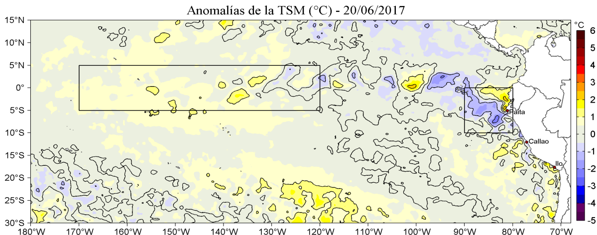
Figura 1. Anomalías de la temperatura superficial del mar ( ^\circ\text{C} ) en el océano Pacífico tropical. Las regiones Niño 3.4 ( 5^\circ\text{N} - 5^\circ\text{S} , 170^\circ\text{W} - 120^\circ\text{W} ) y Niño 1+2 ( 0^\circ - 10^\circ\text{S} , 90^\circ\text{W} - 80^\circ\text{W} ) en los sectores central y oriental del océano, respectivamente, están delimitadas con una línea de color negro. Climatología: 2007-2016. Datos: OSTIA-UKMO-L4-GLOB-v2.0 (UK Met Office, 2012; Donlon et al, 2012) disponible en https://podaac.jpl.nasa.gov/dataset/OSTIA-UKMO-L4-GLOB-v2.0 . Procesamiento: IMARPE.
