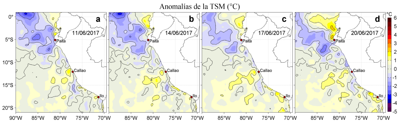
Figura 3. Anomalías de la Temperatura Superficial del Mar ( ^{\circ}\text{C} ) para los días: a) 11, b) 14, c) 17, y d) 20 de junio de 2017. Las anomalías se calcularon respecto de la climatología para el periodo 2007-2016. Datos: OSTIA-UKMO-L4-GLOB-v2.0 (UK Met Office, 2012; Donlon et al, 2012). Procesamiento: LHF/AFIOF/DGIOCC/IMARPE.
