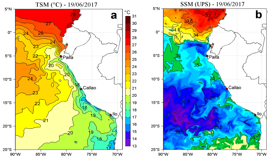
Figura 2. a) Temperatura superficial del mar ( ^{\circ}\text{C} ) y b) Salinidad superficial del mar (UPS) para el 19 de junio. Datos: OSTIA-UKMO-L4-GLOB-v2.0 (UK Met Office, 2012; Donlon et al, 2012) disponible en https://podaac.jpl.nasa.gov/dataset/OSTIA-UKMO-L4-GLOB-v2.0 para (a) y Hybrid Coordinate Ocean Model (HYCOM; Halliwell et al., 1998; 2000; Bleck, 2001) para (b). Procesamiento: AFSR/DGIHSA/IMARPE.
