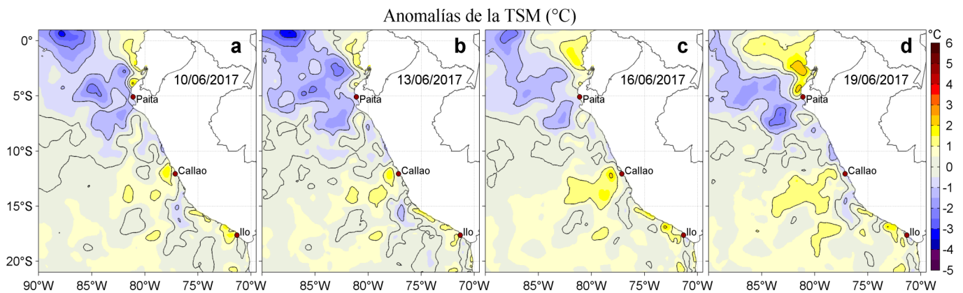
Figura 3. Anomalías de la Temperatura Superficial del Mar ( ^{\circ}\text{C} ) para los días: a) 10, b) 13, c) 16, y d) 19 de junio de 2017. Las anomalías se calcularon respecto de la climatología para el periodo 2007-2016. Datos: OSTIA-UKMO-L4-GLOB-v2.0 (UK Met Office, 2012; Donlon et al, 2012). Procesamiento: LHF/AFIOF/DGIOCC/IMARPE.
