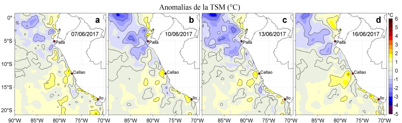
Figura 3. Anomalías de la Temperatura Superficial del Mar ( ^{\circ}\text{C} ) para los días: a) 07, b) 10, c) 13, y d) 16 de junio de 2017. Las anomalías se calcularon respecto de la climatología para el periodo 2007-2016. Datos: OSTIA-UKMO-L4-GLOB-v2.0 (UK Met Office, 2012; Donlon et al, 2012). Procesamiento: LHF/AFIOF/DGIOCC/IMARPE.
