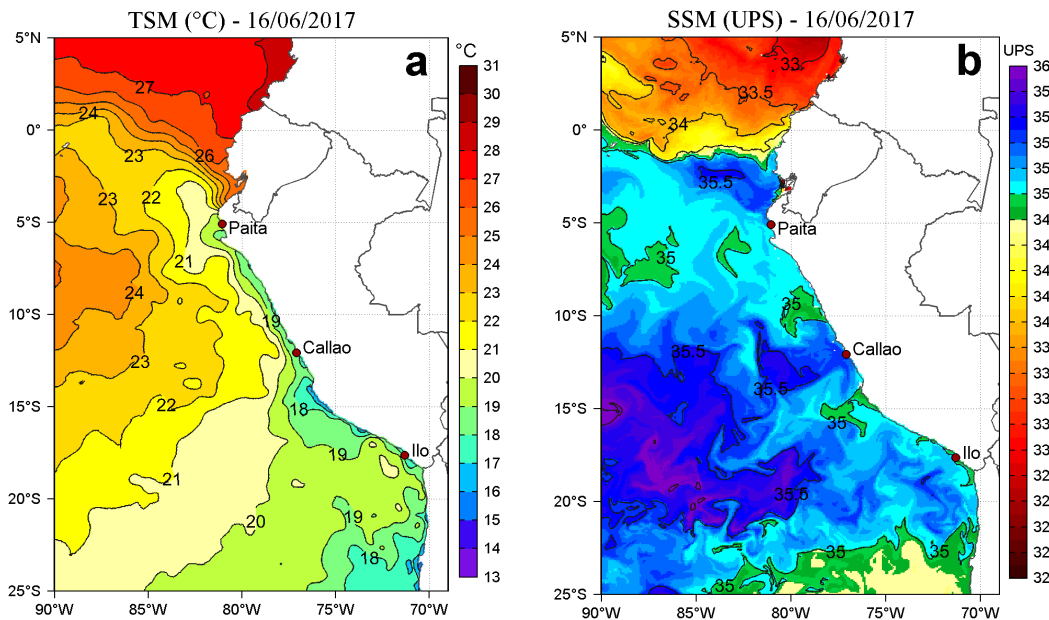
Figura 2. a) Temperatura superficial del mar ( ^{\circ}\text{C} ) y b) Salinidad superficial del mar (UPS) para el 16 de junio. Datos: OSTIA-UKMO-L4-GLOB-v2.0 (UK Met Office, 2012; Donlon et al, 2012) disponible en https://podaac.jpl.nasa.gov/dataset/OSTIA-UKMO-L4-GLOB-v2.0 para (a) y Hybrid Coordinate Ocean Model (HYCOM; Halliwell et al., 1998; 2000; Bleck, 2001) para (b). Procesamiento: AFSR/DGIHSA/IMARPE.
