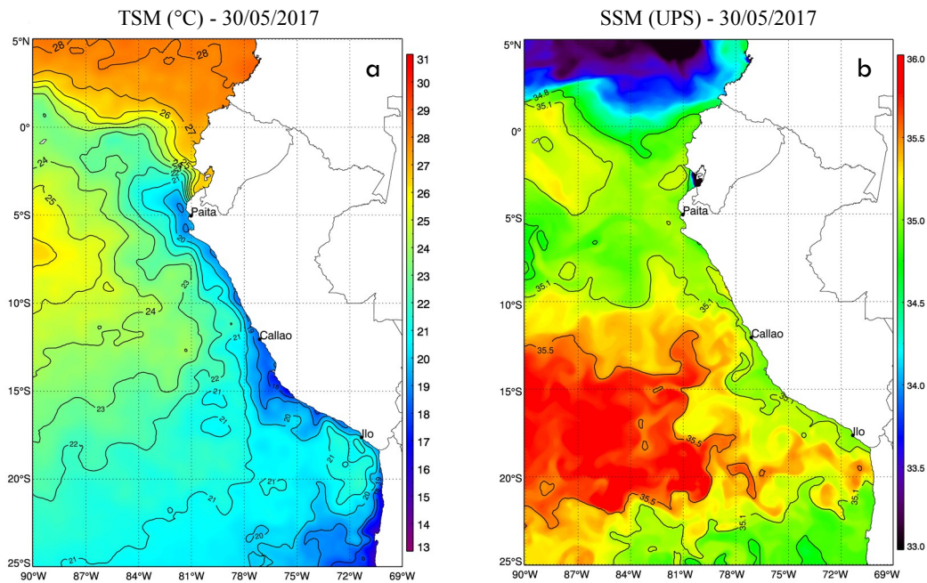
Figura 2. a) Temperatura superficial del mar ( ^{\circ}\text{C} ) y b) Salinidad superficial del mar (UPS) para el 30 de mayo. Datos: OSTIA-UKMO-L4-GLOB-v2.0 (UK Met Office, 2012; Donlon et al, 2012) disponible en https://podaac.jpl.nasa.gov/dataset/OSTIA-UKMO-L4-GLOB-v2.0 para (a) y Hybrid Coordinate Ocean Model (HYCOM; Halliwell et al., 1998; 2000; Bleck, 2001) para (b). Procesamiento: AFSR/DGIHSA/IMARPE.
