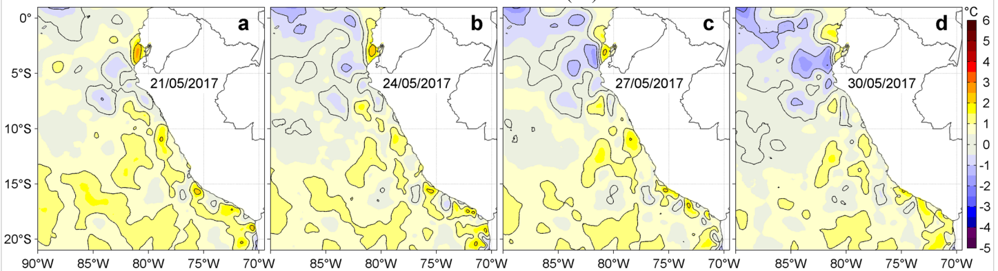
Figura 3. Anomalías de la Temperatura Superficial del Mar ( ^{\circ}\text{C} ) para los días: a) 21, b) 24, c) 27 y d) 30 de mayo de 2017. Las anomalías se calcularon respecto de la climatología para el periodo 2007-2016. Datos: OSTIA-UKMO-L4-GLOB-v2.0 (UK Met Office, 2012; Donlon et al, 2012). Procesamiento: LHF/AFIOF/DGIOCC/IMARPE.
