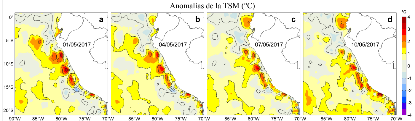
Figura 3. Anomalías de la Temperatura Superficial del Mar ( ^{\circ}\text{C} ) para los días: a) 01, b) 04, c) 07 y d) 10 de mayo de 2017. Las anomalías se calcularon respecto de la climatología para el periodo 2007-2016. Datos: OSTIA-UKMO-L4-GLOB-v2.0 (UK Met Office, 2012; Donlon et al, 2012). Procesamiento: LHF/AFIOF/DGIOCC/IMARPE.
