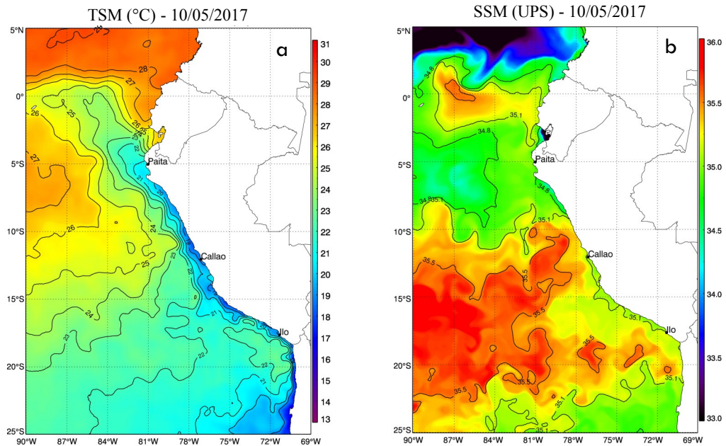
Figura 2. a) Temperatura superficial del mar ( ^{\circ}\text{C} ) y b) Salinidad superficial del mar (UPS) para el 10 de mayo. Datos: OSTIA-UKMO-L4-GLOB-v2.0 (UK Met Office, 2012; Donlon et al, 2012) disponible en https://podaac.jpl.nasa.gov/dataset/OSTIA-UKMO-L4-GLOB-v2.0 ) para (a) y Hybrid Coordinate Ocean Model (HYCOM; Halliwell et al., 1998; 2000; Bleck, 2001) para (b). Procesamiento: AFSR/DGIHSA/IMARPE.
