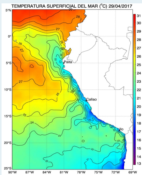
Figura 4. Distribución espacial de la temperatura superficial del mar (°C) en Perú. Datos: OSTIA/PODAAC. Procesamiento: IMARPE.
