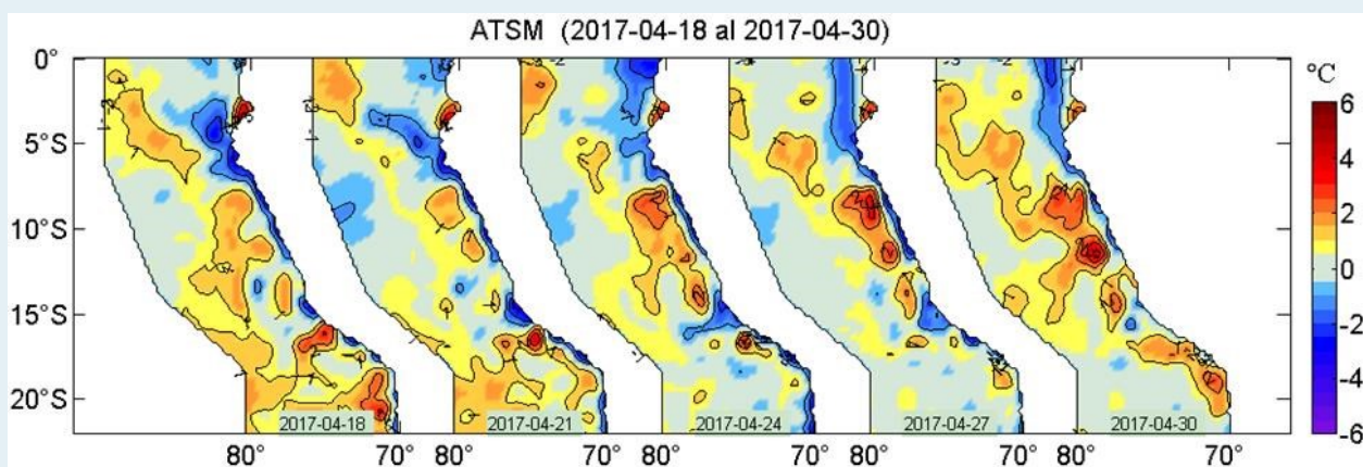
Figura 2. Anomalías de la temperatura superficial del agua (°C) en el mar peruano, cada tres días, entre el 18 y 30 de abril del 2017. Datos: AVHRR Global Reyn_SmithOlv2R (Reynolds, et. al., 2007) de CMB/EMC/NCEP de la NOAA. Procesamiento: IMARPE.
