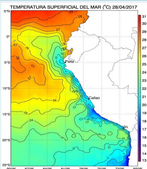
Figura 4. Distribución espacial de la temperatura superficial del mar (°C) en Perú. Datos: OSTIA/PODAAC. Procesamiento: IMARPE.
