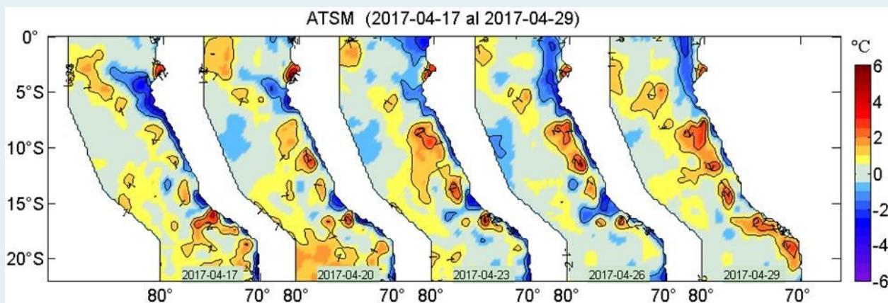
Figura 2. Anomalías de la temperatura superficial del agua (TSM, °C) en el mar peruano, cada tres días, entre el 17 y 29 de abril del 2017. Datos: AVHRR Global Reyn_SmithOiv2R (Reynolds, et. al., 2007) de CMB/EMC/NCEP de la NOAA. Procesamiento: IMARPE.
