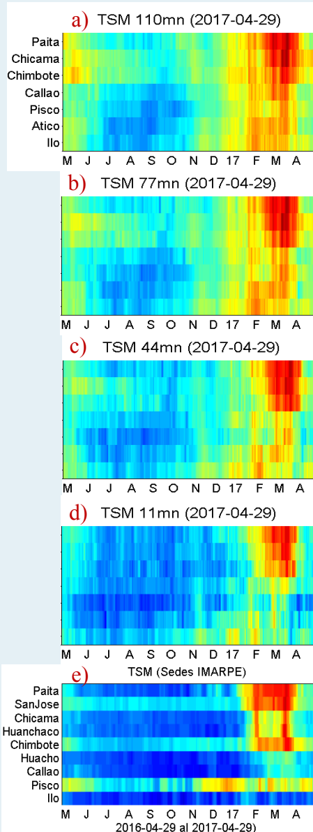
Figura 4. Distribución espacial de la temperatura superficial del mar (°C) en Perú. Datos: OSTIA/PODAAC. Procesamiento: IMARPE.
