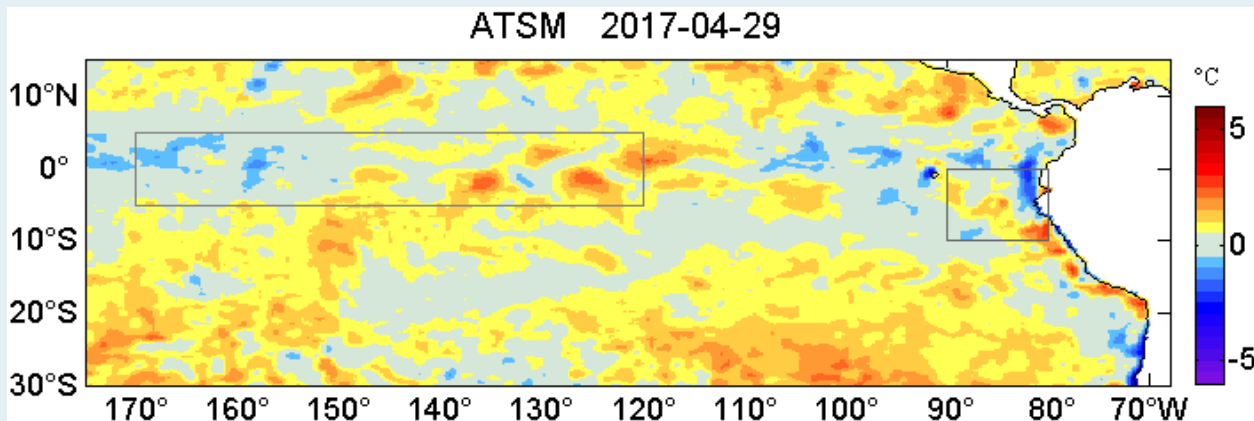
Figura 1. Anomalías de la temperatura superficial del mar (ATSM, °C) en el océano Pacífico tropical. Las regiones Niño 3.4 y Niño 1+2 en los sectores central y oriental del océano, respectivamente, están delimitadas con una línea de color negro. Datos: AVHRR Global Reyn_SmithOiv2R (Reynolds, et. al., 2007) de CMB/EMC/NCEP de la Administración Nacional del Océano y la Atmósfera (NOAA, según sus siglas en inglés). Procesamiento: IMARPE.
