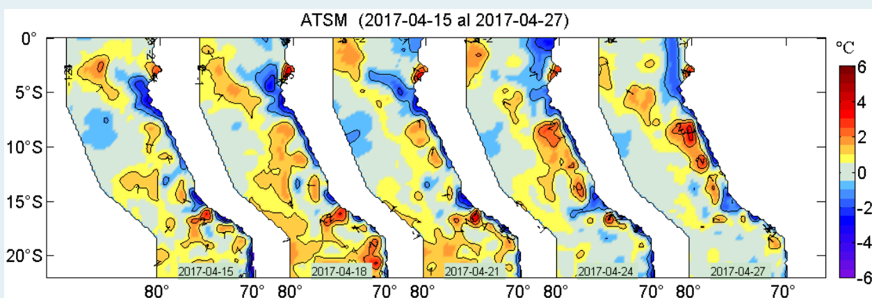
Figura 2. Anomalías de la temperatura superficial del agua (°C) en el mar peruano, cada tres días, entre el 15 y 27 de abril del 2017. Datos: AVHRR Global Reyn_SmithOlv2R (Reynolds, et. al., 2007) de CMB/EMC/NCEP de la NOAA. Procesamiento: IMARPE.
