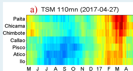
Figura 4. Distribución espacial de la temperatura superficial del mar (°C) en Perú. Datos: OSTIA/PODAAC. Procesamiento: IMARPE.
