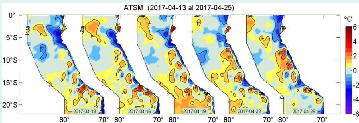
Figura 2. Anomalías de la temperatura superficial del agua (°C) en el mar peruano, cada tres días, entre el 13 y 25 de abril del 2017. Datos: AVHRR Global Reyn_SmithOlv2R (Reynolds, et. al., 2007) de CMB/EMC/NCEP de la NOAA. Procesamiento: IMARPE.
