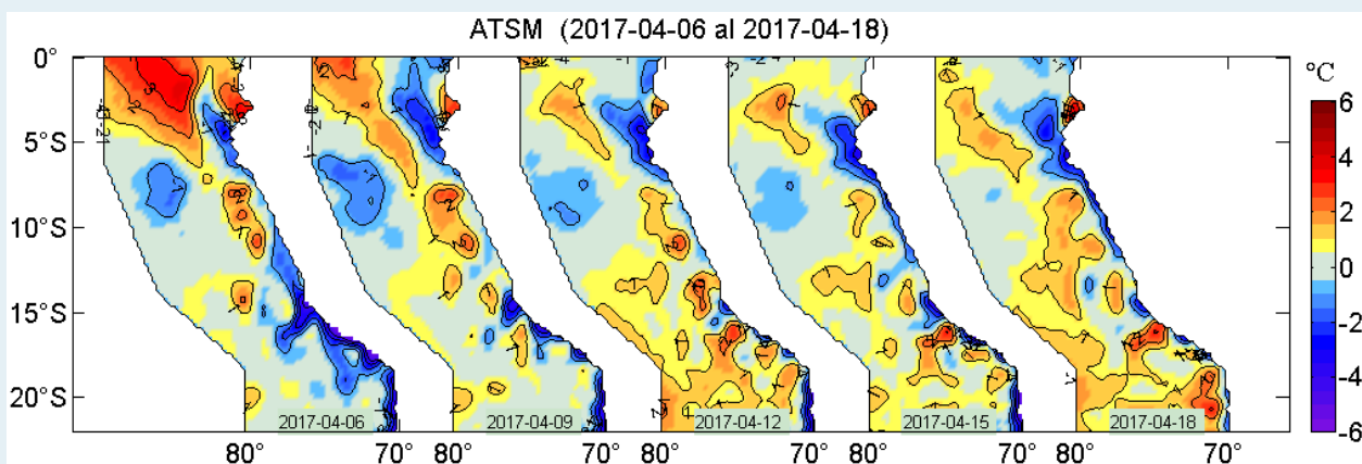
Figura 2. Anomalías de la temperatura superficial del agua (°C) en el mar peruano, cada tres días, entre el 06 y 18 de abril del 2017. Datos: AVHRR Global Reyn_SmithOlv2R (Reynolds, et. al., 2007) de CMB/EMC/NCEP de la NOAA. Procesamiento: IMARPE.
