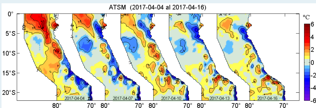
Figura 2. Anomalías de la temperatura superficial del agua (°C) en el mar peruano, cada tres días, entre el 04 y 16 de abril del 2017. Datos: AVHRR Global Reyn_SmithOlv2R (Reynolds, et. al., 2007) de CMB/EMC/NCEP de la NOAA. Procesamiento: IMARPE.
