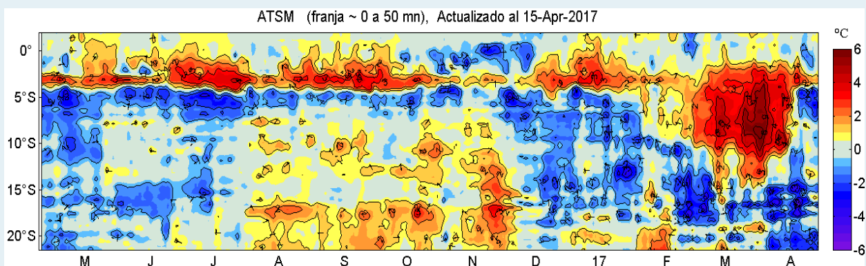
Figura 3. Evolución latitudinal de las anomalías promedio diarias de la temperatura superficial del mar (°C) para la franja de ~50 mn adyacentes al litoral peruano. Datos: AVHRR Global Reyn_SmithO1v2R (Reynolds, et. al., 2007) de CMB/EMC/NCEP de la NOAA. Procesamiento: IMARPE.
