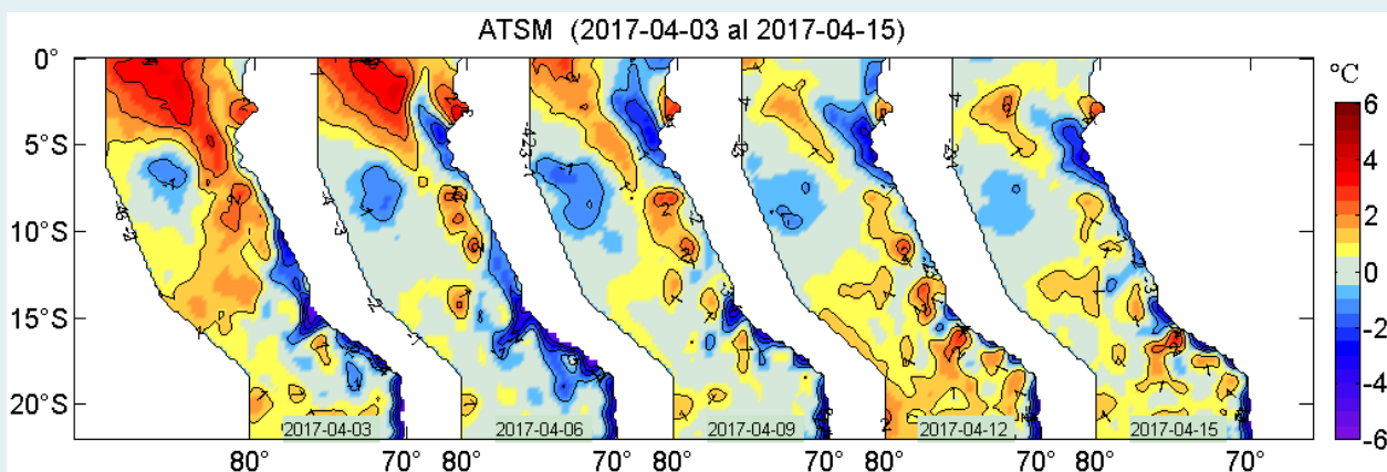
Figura 2. Anomalías de la temperatura superficial del agua (°C) en el mar peruano, cada tres días, entre el 03 y 15 de abril del 2017. Datos: AVHRR Global Reyn_SmithO1v2R (Reynolds, et. al., 2007) de CMB/EMC/NCEP de la NOAA. Procesamiento: IMARPE.
