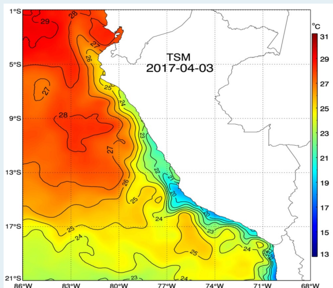
Figura 4. Distribución espacial de la temperatura superficial del mar (°C) en Perú. Datos: OSTIA/PODAAC. Procesamiento: IMARPE.
