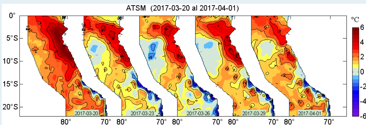
Figura 2. Anomalías de la temperatura superficial del agua (°C) en el mar peruano, cada tres días, entre el 20 de marzo y 01 de abril del 2017. Datos: AVHRR Global Reyn_SmithOlv2R (Reynolds, et. al., 2007) de CMB/EMC/NCEP de la NOAA. Procesamiento: IMARPE.
