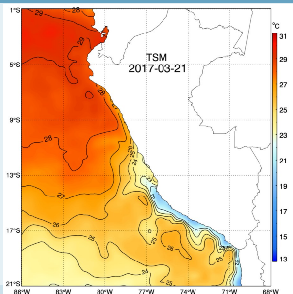
Figura 4. Distribución espacial de la temperatura superficial del mar (°C) peruano. Datos: OSTIA. Procesamiento: IMARPE.
