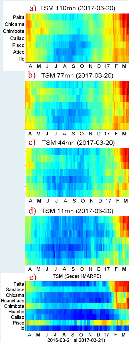
Figura 4. Distribución espacial de la temperatura superficial del mar (°C) peruano. Datos: OSTIA. Procesamiento: IMARPE.
