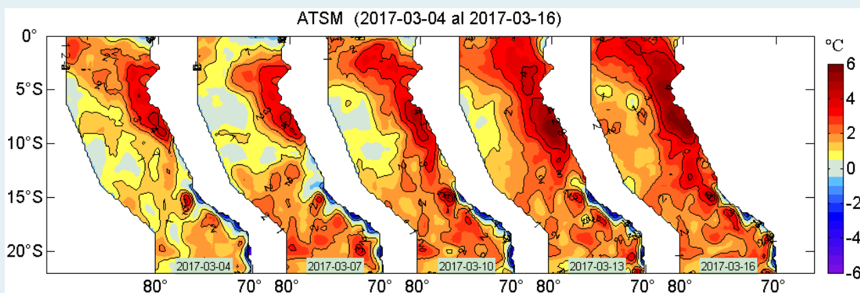
Figura 2. Anomalías de la temperatura superficial del agua (°C) en el mar peruano, cada tres días, entre el 04 y 16 de marzo del 2017. Datos: AVHRR Global Reyn_SmithOlv2R (Reynolds, et. al., 2007) de CMB/EMC/NCEP de la NOAA. Procesamiento: IMARPE.
