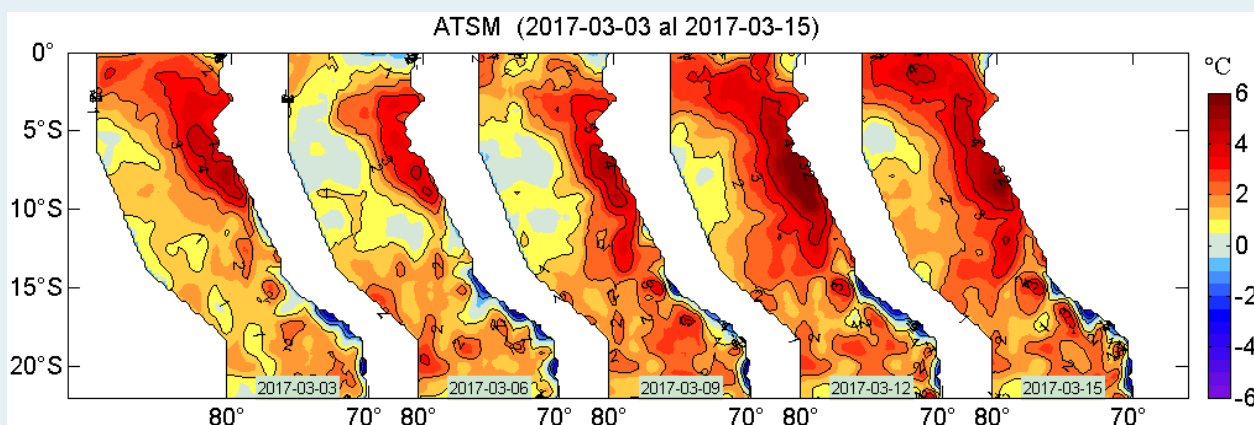
Figura 2. Anomalías de la temperatura superficial del agua (°C) en el mar peruano, cada tres días, entre el 03 y 15 de marzo del 2017. Datos: AVHRR Global Reyn_SmithOlv2R (Reynolds, et. al., 2007) de CMB/EMC/NCEP de la NOAA. Procesamiento: IMARPE.
