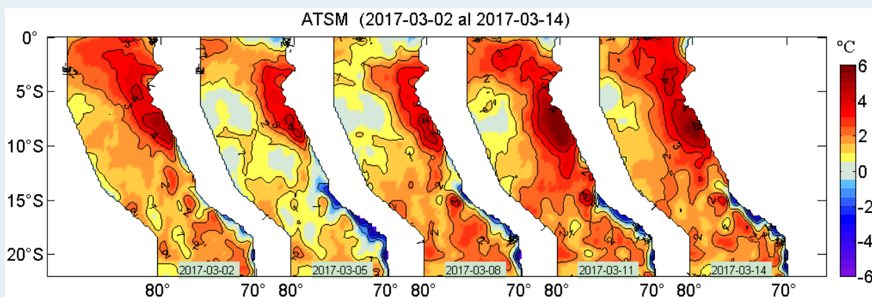
Figura 2. Anomalías de la temperatura superficial del agua (°C) en el mar peruano, cada tres días, entre el 02 y 14 de marzo del 2017. Datos: AVHRR Global Reyn_SmithOlv2R (Reynolds, et. al., 2007) de CMB/EMC/NCEP de la NOAA. Procesamiento: IMARPE.
