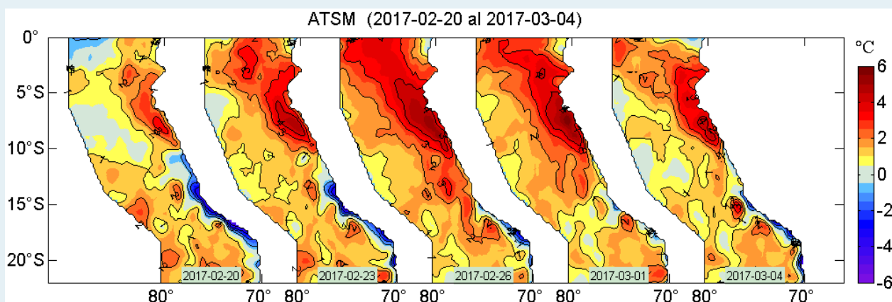
Figura 2. Anomalías de la temperatura superficial del agua (°C) en el mar peruano, cada tres días, entre el 20 de febrero y 04 de marzo del 2017. Datos: AVHRR Global Reyn_SmithOlv2R (Reynolds, et. al., 2007) de CMB/EMC/NCEP de la NOAA. Procesamiento: IMARPE.
