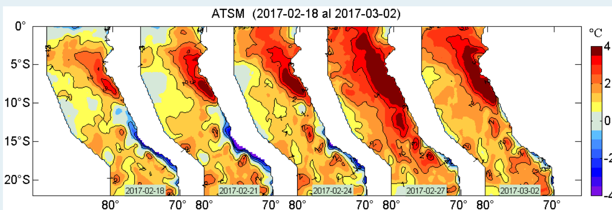
Figura 2. Anomalías de la temperatura superficial del agua (°C) en el mar peruano, cada tres días, entre el 18 de febrero y 02 de marzo del 2017. Datos: AVHRR Global Reyn_SmithOiv2R (Reynolds, et. al., 2007) de CMB/EMC/NCEP de la NOAA. Procesamiento: IMARPE.
