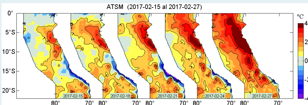
Figura 2. Anomalías de la temperatura superficial del agua (°C) en el mar peruano, cada tres días, entre el 15 y 27 de febrero del 2017. Datos: AVHRR Global Reyn_SmithOlv2R (Reynolds, et. al., 2007) de CMB/EMC/NCEP de la NOAA. Procesamiento: IMARPE.
