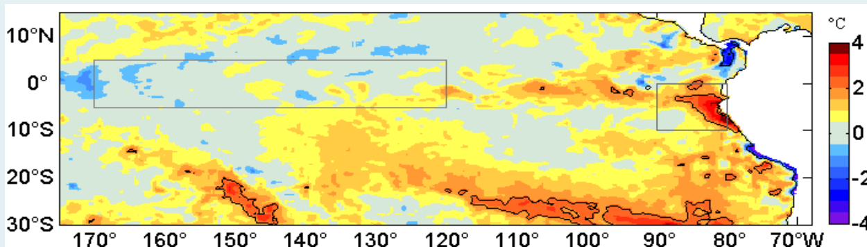
Figura 1. Anomalías de la temperatura superficial del mar (°C) en el océano Pacífico tropical. Las regiones Niño 3.4 y Niño 1+2 en los sectores central y oriental del océano, respectivamente, están delimitadas con una línea de color negro. Datos: AVHRR Global Reyn_SmithOlv2R (Reynolds, et. al., 2007) de CMB/EMC/NCEP de la Administración Nacional del Océano y la Atmósfera (NOAA, según sus siglas en inglés). Procesamiento: IMARPE.
