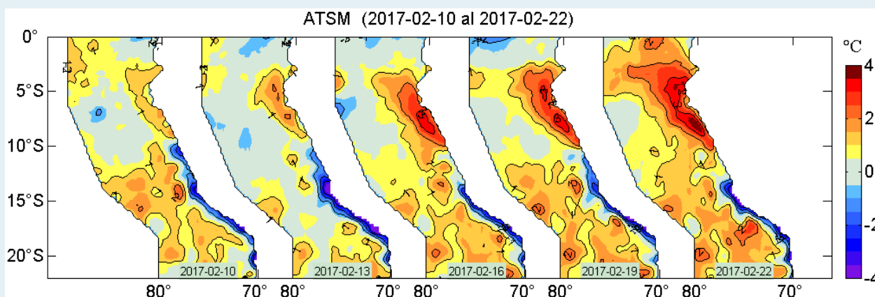
Figura 2. Anomalías de la temperatura superficial del agua (°C) en el mar peruano, cada tres días, entre el 10 y 22 de febrero del 2017. Datos: AVHRR Global Reyn_SmithOlv2R (Reynolds, et. al., 2007) de CMB/EMC/NCEP de la NOAA. Procesamiento: IMARPE.
