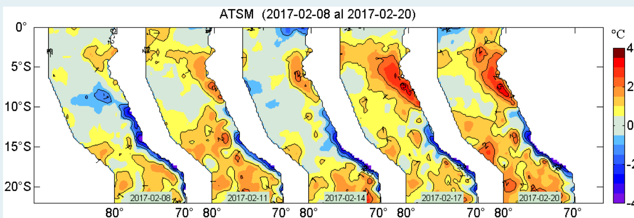
Figura 2. Anomalías de la temperatura superficial del agua (°C) en el mar peruano, cada tres días, entre el 08 y 20 de febrero del 2017. Datos: AVHRR Global Reyn_SmithOlv2R (Reynolds, et. al., 2007) de CMB/EMC/NCEP de la NOAA. Procesamiento: IMARPE.
