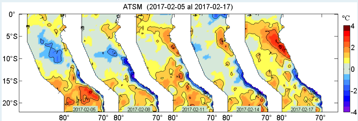
Figura 2. Anomalías de la temperatura superficial del agua (°C) en el mar peruano, cada tres días, entre el 05 y 17 de febrero del 2017. Datos: AVHRR Global Reyn_SmithOlv2R (Reynolds, et. al., 2007) de CMB/EMC/NCEP de la NOAA. Procesamiento: IMARPE.
