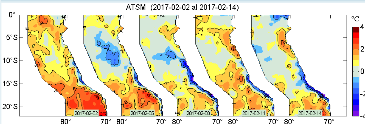
Figura 2. Anomalías de la temperatura superficial del agua (°C) en el mar peruano, cada tres días, entre el 02 y 14 de febrero del 2017. Datos: AVHRR Global Reyn_SmithOiv2R (Reynolds, et. al., 2007) de CMB/EMC/NCEP de la NOAA. Procesamiento: IMARPE.
