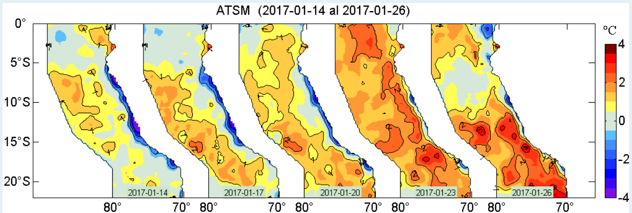
Figura 2. Anomalías de la temperatura superficial del agua (°C) en el mar peruano, cada tres días, entre el 14 y 26 de enero del 2017. Datos: AVHRR Global Reyn_SmithOiv2R (Reynolds, et. al., 2007) de CMB/EMC/NCEP de la NOAA. Procesamiento: IMARPE.
