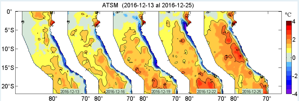
Figura 2. Anomalías de la temperatura superficial del agua (°C) en el mar peruano, cada tres días, entre el 13 y 25 de diciembre del 2016. Datos: AVHRR Global Reyn_SmithOiv2R (Reynolds, et. al., 2007) de CMB/EMC/NCEP de la NOAA. Procesamiento: IMARPE.
