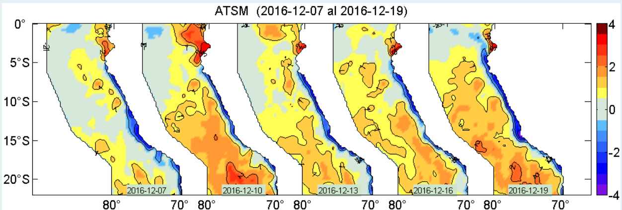
Figura 2. Anomalías de la temperatura superficial del agua (°C) en el mar peruano, cada tres días, entre el 07 y 19 de diciembre del 2016. Datos: AVHRR Global Reyn_SmithOiv2R (Reynolds, et. al., 2007) de CMB/EMC/NCEP de la NOAA. Procesamiento: IMARPE.
