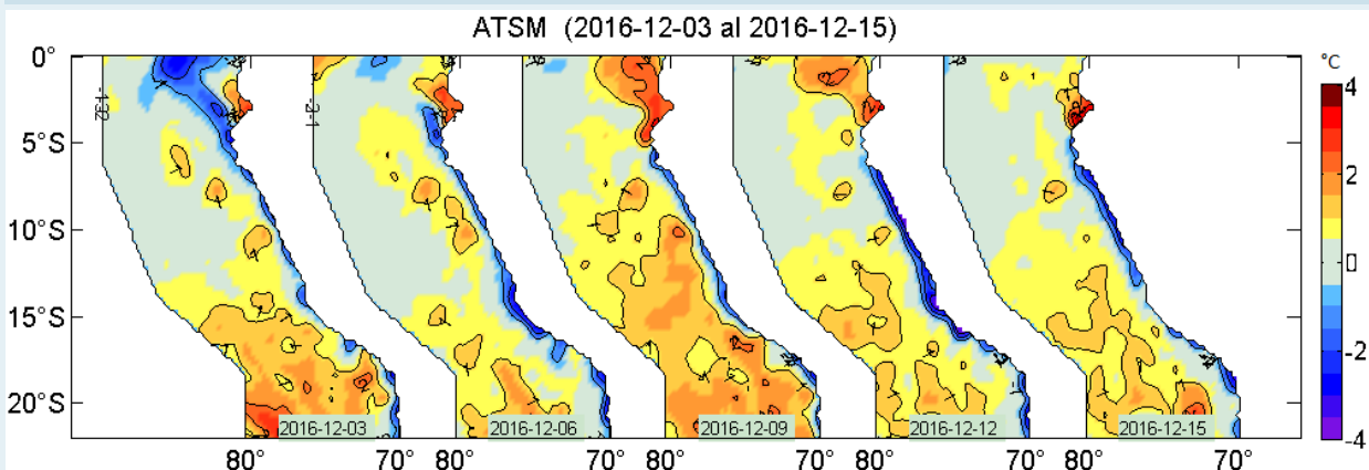
Figura 2. Anomalías de la temperatura superficial del agua (°C) en el mar peruano, cada tres días, entre el 03 y 15 de diciembre del 2016. Datos: AVHRR Global Reyn_SmithOIv2R (Reynolds, et. al., 2007) de CMB/EMC/NCEP de la NOAA. Procesamiento: IMARPE.
